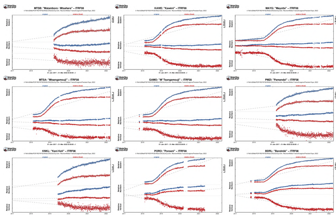
Figure 9 : Déplacements (en cm) enregistrés sur les 9 stations GPS localisées à Mayotte (MTSB, KAWE, MAYG, MTSA, GAMO, PMZI, KNKL, PORO, BDRL) entre le 1 er janvier 2017 et 31 mars 2022 pour visualiser une longue série temporelle anté-crise. En bleu les données brutes, en rouge les données corrigées du mouvement de la plaque. Les stations sont présentées dans un ordre géographique ; du nord au sud (de haut en bas) et d'ouest en est (de gauche à droite). Post-traitement de ces données réalisé par l'IPGP (©OVPF-IPGP / REVOSIMA).
