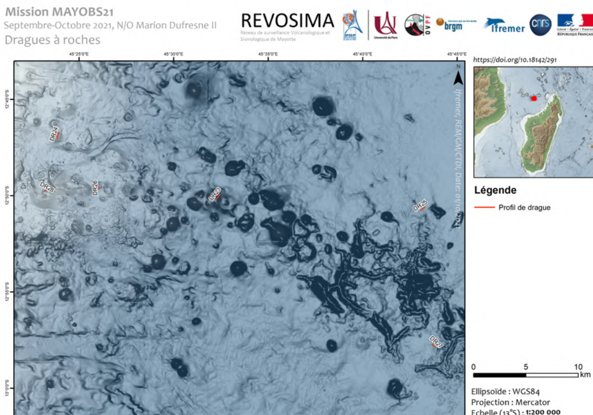
Figure 11 : Localisation des dragages effectués lors de la campagne MAYOBS21 (©REVOSIMA).
