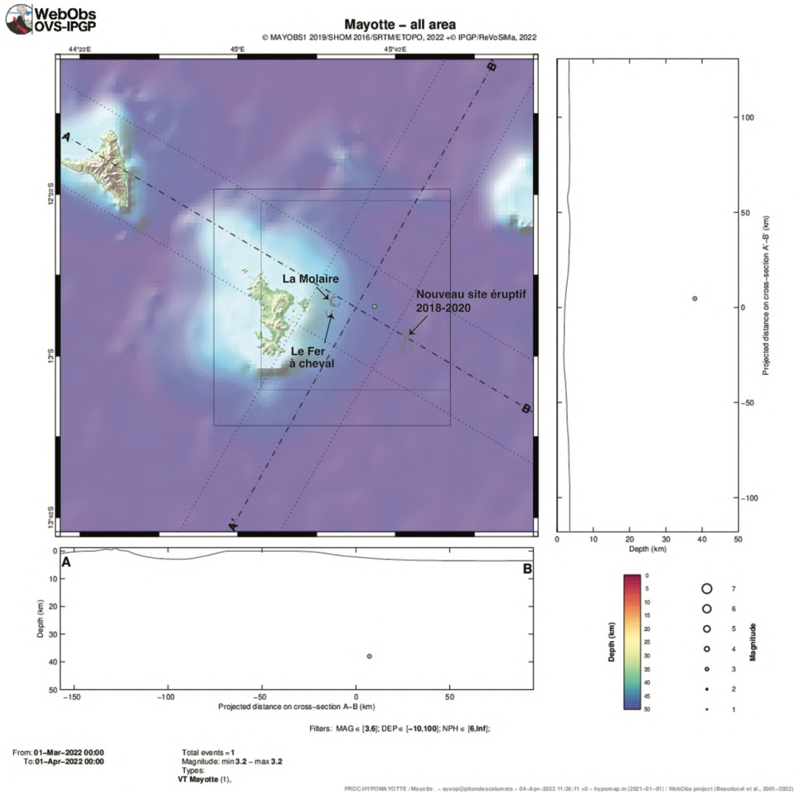
Figure 1c : Carte de localisation des épicentres ( \pm 5 km) des séismes volcano-tectoniques (VT) de magnitude M \geq 3 entre le 1 er et le 31 mars 2022 enregistrés avec les réseaux sismiques à terre (IPGP-IFREMER-CNRS-BRGM-BCSF-RENASS, ITES). Sont aussi représentées une projection des hypocentres des séismes le long de coupes transverses et axiales le long de la ride montrant la localisation estimée en profondeur (la précision varie entre \pm 5 km et \pm 15 km) des séismes en fonction de la magnitude (taille des symboles) et de la date (échelle temporelle de couleur). Les structures volcaniques de la zone dite de « La Molaire », du « Fer à cheval » sont indiquées en gris tout comme les coulées de lave du site éruptif. De nombreux points de sortie de panaches de fluides dans la colonne d'eau ont été identifiés dans la structure du Fer à Cheval avec une signature géochimique magmatique (voir section Géochimie des fluides). © OVPF-IPGP, BRGM, IFREMER, CNRS, BCSF-RENASS, ITES / REVOSIMA).
