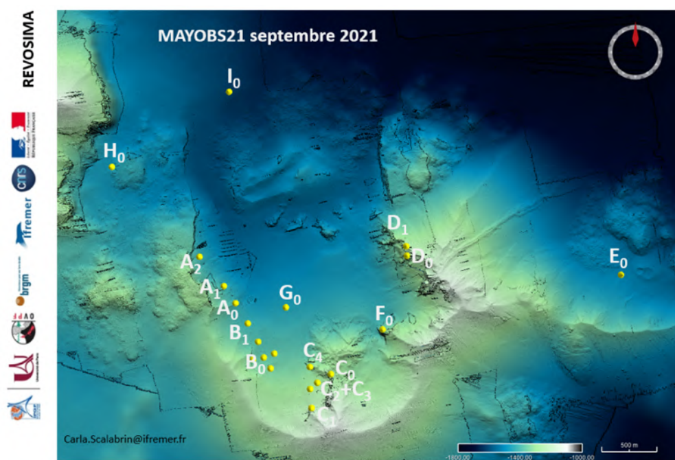
Figure 10 : Répartition des sites actifs (panaches acoustiques) dans la zone du Fer à Cheval (©REVOSIMA).
