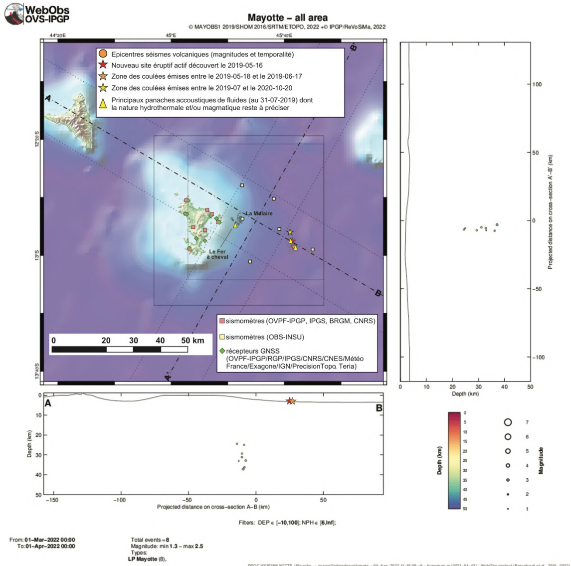
Figure 1b : Carte des épicentres ( \pm 5 km) des séismes longue période (LP) localisés avec les réseaux sismiques à terre (IPGP-IFREMER-CNRS-BRGM-BCSF-RENASS, ITES) entre le 1 er et 31 mars 2022 (échelle temporelle de couleur). Sont aussi représentées une projection des hypocentres des séismes le long de coupes transverses et axiales le long de la ride montrant la localisation estimée en profondeur (la précision varie entre \pm 5 km et \pm 15 km) des séismes en fonction de la magnitude (taille des symboles et de la date (échelle temporelle de couleur)). La localisation approximative des panaches acoustiques identifiés pendant les campagnes océanographiques (MD220-MAYOBS1, MD221-MAYOBS2, MD222-MAYOBS3, MD223-MAYOBS4, MAYOBS15, MAYOBS17) et dont la nature hydrothermale et/ou magmatique reste à préciser, est indiquée par des triangles jaunes, l'étoile rouge indique le site éruptif nouvellement identifié le 16 mai 2019, l'étoile orange la zone des coulées émises entre le 18/05/2019 et le 17/06/2019 et l'étoile jaune la zone des coulées émises entre juillet 2019 et le 18/01/2021. Les structures volcaniques de la zone dite de « La Molaire » sont indiquées en gris tout comme les coulées de lave du site éruptif. Les stations sismiques du réseau terrestre, les sismomètres fond de mer (OBS) et les stations de positionnement par satellite GPS sont indiquées par des symboles (voir légende). (©OVPF-IPGP, BRGM, IFREMER, CNRS, BCSF-RENASS, ITES / REVOSIMA).
