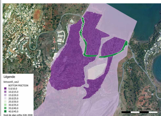
Illustration 18: carte des coefficients de rugosité - secteur 2
