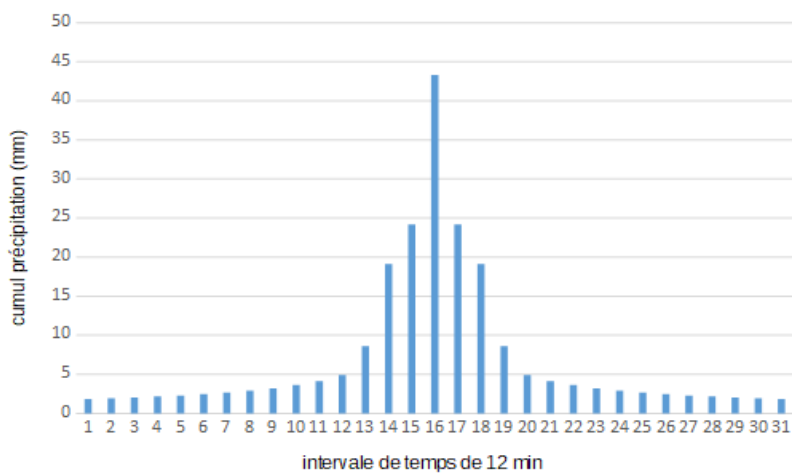
Illustration 6: pluie de projet – T10 ans
