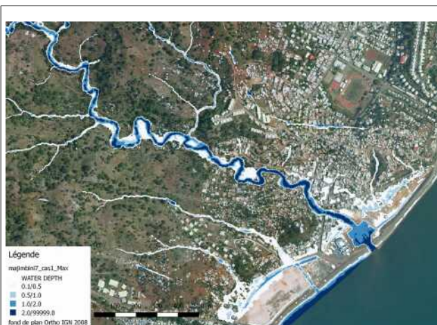
Illustration 39: secteur 4 – Qfreq – Hmax
