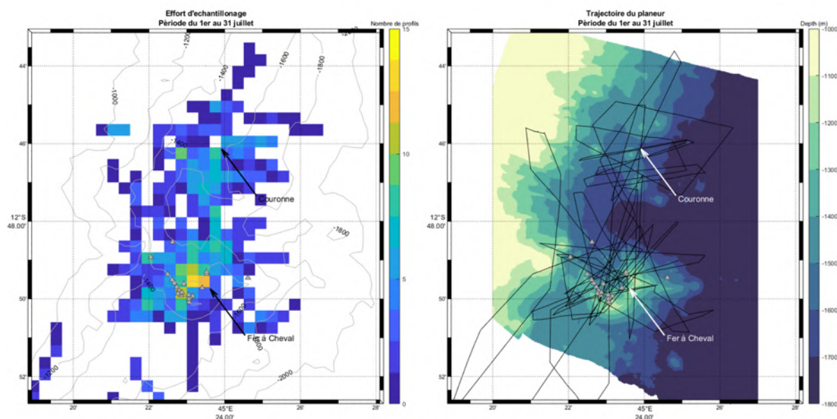
Figure 16 : (gauche) Carte illustrant l'effort d'échantillonnage à partir du nombre de profils acquis par le SeaExplorer dans des rectangles de 0.5 km 2 , entre le 1 er et le 31 juillet 2022. (droite) Carte des trajectoires du planeur sous-marin sur la même période. Les triangles sont les sites actifs d'émission de fluides identifiés avec le sondeur multifaisceaux coque pendant les campagnes MAYOBS du REVOSIMA (DOI 10.12770/070818f6-6520-49e4-bafd-9d4d0609bf7d) et validés par des observations visuelles in situ avec le ROV VICTOR lors de la campagne GEOFLAMME (DOI 10.17600/18001297).
