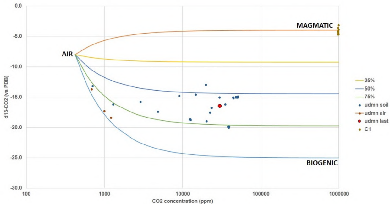
Figure 12 : Variations isotopiques du carbone ( \delta^{13}\text{C}\text{-CO}_2 ) du CO 2 dans l'air et dans les gaz du sol à la station UDMN. La composition du pôle magmatique est fixée à -4.0 per mil (signature des bullages du site C1 – estran de l'aéroport).
