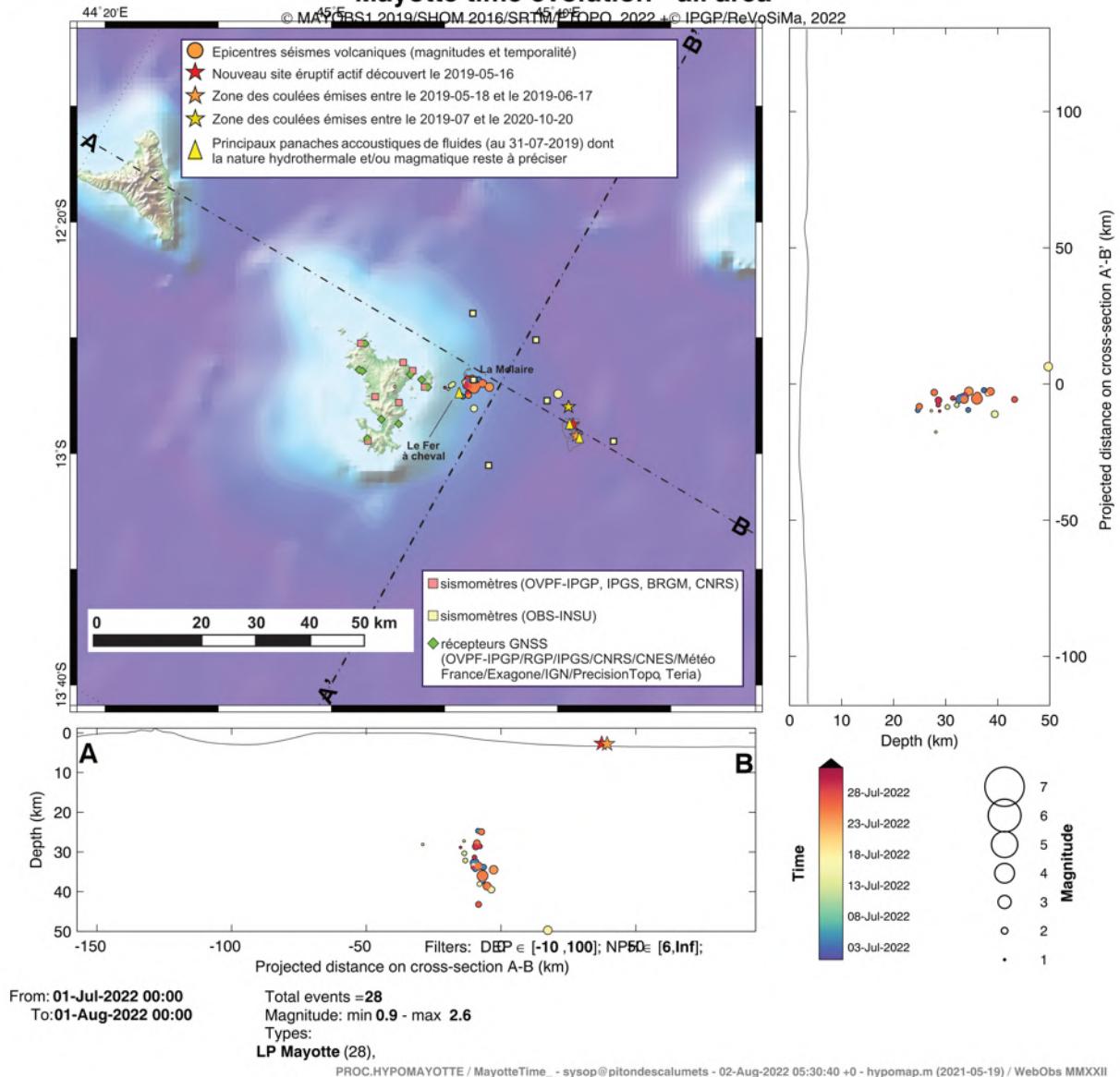
Figure 1b : Carte des épicentres ( \pm 5 km) des séismes longue période (LP) localisés avec les réseaux sismiques à terre (IPGP-IFREMER-CNRS-BRGM-BCSF-RENASS, ITES) entre le 1 er et 31 juillet 2022 (échelle temporelle de couleur). Sont aussi représentées une projection des hypocentres des séismes le long de coupes transverses et axiales le long de la ride montrant la localisation estimée en profondeur (la précision varie entre \pm 5 km et \pm 15 km) des séismes en fonction de la magnitude (taille des symboles et de la date (échelle temporelle de couleur)). La localisation approximative des panaches acoustiques identifiés pendant les campagnes océanographiques (MD220-MAYOBS1, MD221-MAYOBS2, MD222-MAYOBS3, MD223-MAYOBS4, MAYOBS15, MAYOBS17) et dont la nature hydrothermale et/ou magmatique reste à préciser, est indiquée par des triangles jaunes, l'étoile rouge indique le site éruptif nouvellement identifié le 16 mai 2019, l'étoile orange la zone des coulées émises entre le 18/05/2019 et le 17/06/2019 et l'étoile jaune la zone des coulées émises entre juillet 2019 et le 18/01/2021. Les structures volcaniques de la zone dite de « La Molaière » sont indiquées en gris tout comme les coulées de lave du site éruptif. Les stations sismiques du réseau terrestre, les sismomètres fond de mer (OBS) et les stations de positionnement par satellite GPS sont indiquées par des symboles (voir légende). (©OVPF-IPGP, BRGM, IFREMER, CNRS, BCSF-RENASS, ITES / REVOSIMA).
