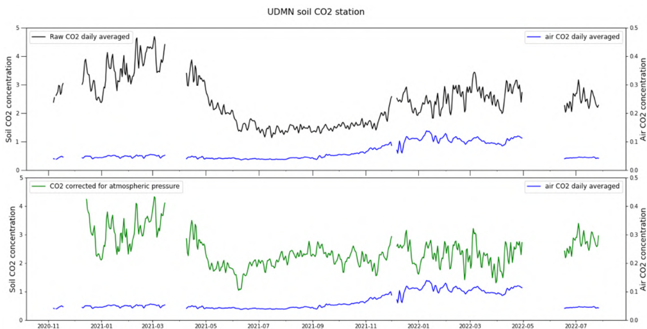
Figure 11 : Concentration en \text{CO}_2 dans le sol à la station permanente UDMN. Comparaison entre les données brutes (noir) et les données corrigées de l'influence de la pression atmosphérique (vert). Bleu : concentration dans l'air (1 m au-dessus du sol). Les variations de concentrations dans l'air sont liées à l'activité biogénique (©OVPF-IPGP / REVOSIMA).
