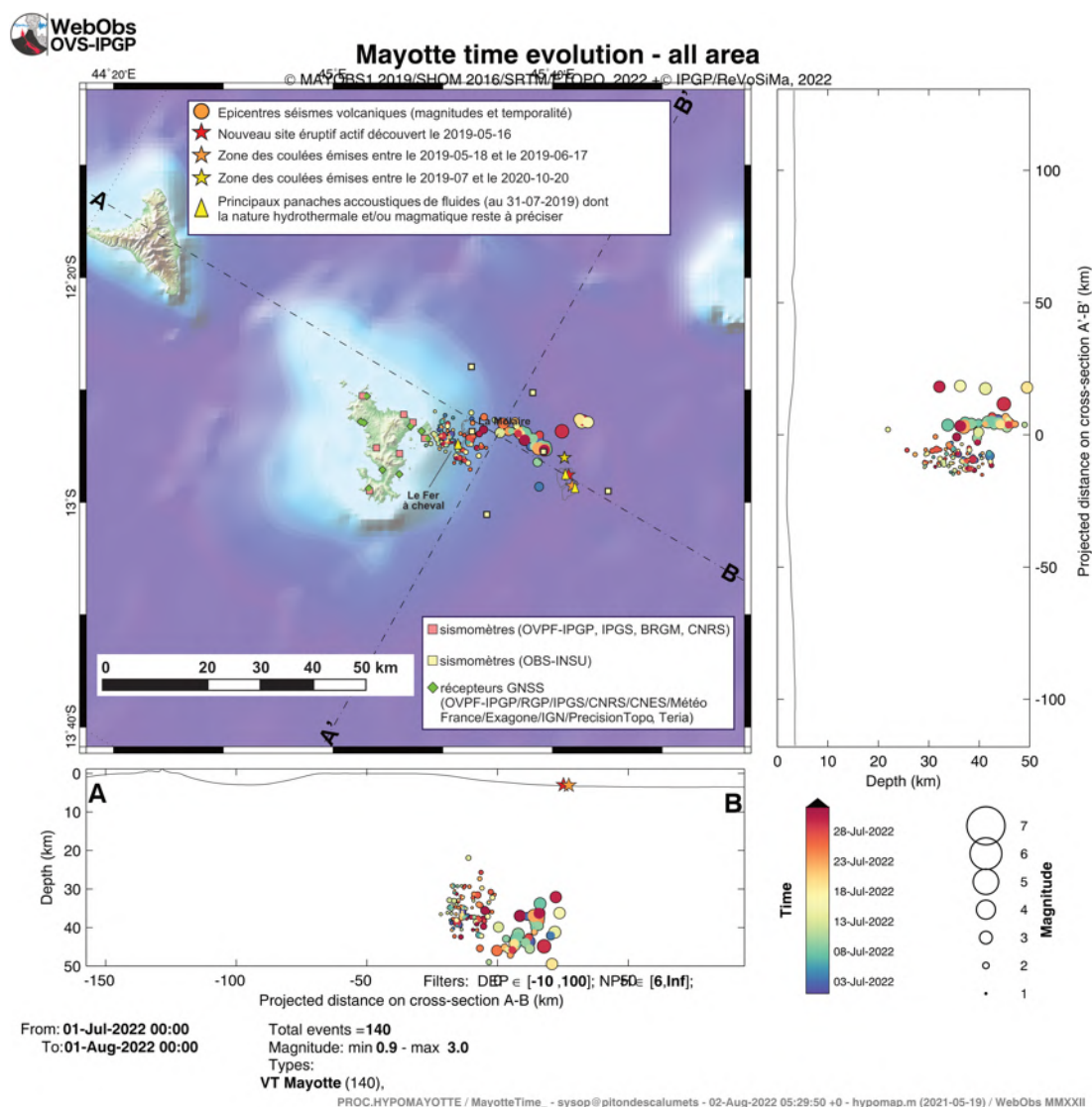
Figure 1a : Carte des épicentres ( \pm 5 km) des séismes volcaniques (VT) localisés avec les réseaux sismiques à terre (IPGP-IFREMER-CNRS-BRGM-BCSF-RENASS, ITES) entre le 1 er et 31 juillet 2022 (échelle temporelle de couleur). Sont aussi représentées une projection des hypocentres des séismes le long de coupes transverses et axiales le long de la ride montrant la localisation estimée en profondeur (la précision varie entre \pm 5 km et \pm 15 km) des séismes en fonction de la magnitude (taille des symboles et de la date (échelle temporelle de couleur)). La localisation approximative des panaches acoustiques identifiés pendant les campagnes océanographiques (MD220-MAYOBS1, MD221-MAYOBS2, MD222-MAYOBS3, MD223-MAYOBS4, MAYOBS15, MAYOBS17) et dont la nature hydrothermale et/ou magmatique reste à préciser, est indiquée par des triangles jaunes, l'étoile rouge indique le site éruptif nouvellement identifié le 16 mai 2019, l'étoile orange la zone des coulées émises entre le 18/05/2019 et le 17/06/2019 et l'étoile jaune la zone des coulées émises entre juillet 2019 et le 18/01/2021. Les structures volcaniques de la zone dite de « La Couronne » sont indiquées en grisé tout comme les coulées de lave du site éruptif. Les stations sismiques du réseau terrestre, les sismomètres fond de mer (OBS) et les stations de positionnement par satellite GPS sont indiquées par des symboles (voir légende). (©OVPF-IPGP, BRGM, IFREMER, CNRS, BCSF-RENASS, ITES / REVOSIMA).
