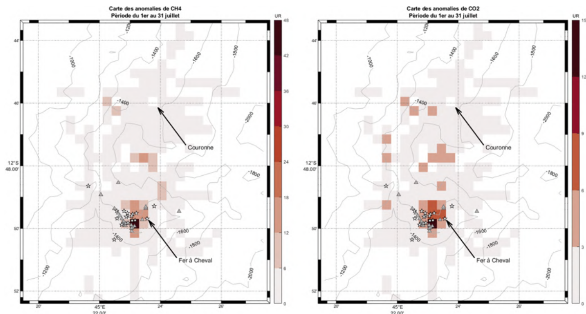
Figure 17 : Carte des anomalies en \text{CH}_4 (gauche) et \text{CO}_2 (droite) dissous mesurées entre 900 et 1000 m de profondeur par le planeur sous-marin entre le 1 er et le 31 juillet. L'échelle de couleur correspond à l'anomalie maximale en gaz dissous exprimée en unité relative dans des rectangles de 0.5 km 2 . Sont aussi représentées par des étoiles les localisations des panaches acoustiques observés entre 900 et 1000 m de profondeur par le planeur sous-marin entre le 1 er et le 31 juillet 2022. Les triangles sont les sites actifs d'émission de fluides identifiés avec le sondeur multifaisceaux coque pendant les campagnes MAYOBS du REVOSIMA (DOI 10.12770/070818f6-6520-49e4-bafd-9d4d0609bf7d) et validés par des observations visuelles in situ avec le ROV VICTOR lors de la campagne GEOFLAMME (DOI 10.17600/18001297).
