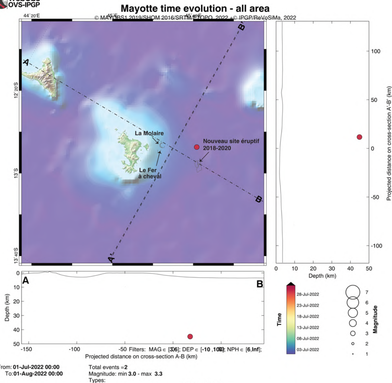
Figure 1c : Carte de localisation des épicentres ( \pm 5 km) des séismes volcano-tectoniques (VT) de magnitude M \geq 3 entre le 1 er et le 31 juillet 2022 enregistrés avec les réseaux sismiques à terre (IPGP-IFREMER-CNRS-BRGM-BCSF-RENASS, ITES). Sont aussi représentées une projection des hypocentres des séismes le long de coupes transverses et axiales le long de la ride montrant la localisation estimée en profondeur (la précision varie entre \pm 5 km et \pm 15 km) des séismes en fonction de la magnitude (taille des symboles) et de la date (échelle temporelle de couleur). Les structures volcaniques de la zone dite de « La Molaire », du « Fer à cheval » sont indiquées en grisé tout comme les coulées de lave du site éruptif. De nombreux points de sortie de panaches de fluides dans la colonne d'eau ont été identifiés dans la structure du Fer à Cheval avec une signature géochimique magmatique (voir section Géochimie des fluides). © OVPF-IPGP, BRGM, IFREMER, CNRS, BCSF-RENASS, ITES / REVOSIMA).
