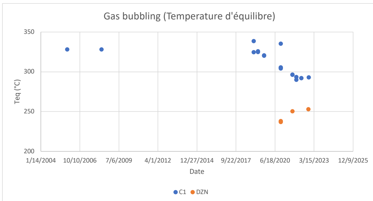
Figure 14 : Température d'équilibre des fluides au sein du système hydrothermal. La température d'équilibre entre le CO 2 et le CH 4 dans le système hydrothermal est estimée à l'aide de l'équation de Guggenbach 1992.
