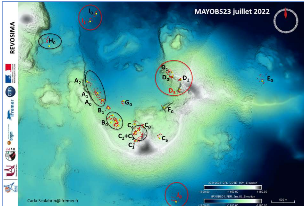
Figure 16 : Localisation des sites actifs d'émission de fluides sur la zone du Fer à Cheval à partir des panaches acoustiques identifiés pendant la campagne MD239-MAYOBS23 et les campagnes de surveillance MAYOBS précédentes et de recherche (SISMAORE, GEOFLAMME, SCRATCH). Les sites labélisés en rouge (D3, I1 et J0) ont été observés pour la première fois pendant la campagne MAYOBS23 en juillet 2022. Les zones actives entourées présentent une augmentation de la surface ou de l'intensité des sites en juillet 2022 par rapport aux campagnes précédentes (H0, I0+I1, A0+A1+A2, B0, C1+C2+C3, D0+D1) (©REVOSIMA).
