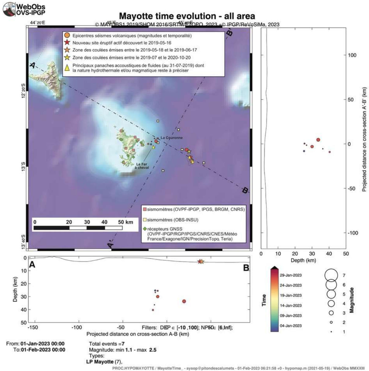
Figure 1b : Carte des épicentres ( \pm 5 km) des séismes longue période (LP) localisés avec les réseaux sismiques à terre (IPGP -CNRS-BRGM-BCSF-RENAISS, ITES) entre le 1 er et 31 janvier 2023 (échelle temporelle de couleur). Sont aussi représentées une projection des hypocentres des séismes le long de coupes transversales et axiales le long de la ride montrant la localisation estimée en profondeur (la précision varie entre \pm 5 km et \pm 15 km) des séismes en fonction de la magnitude (taille des symboles) et de la date (échelle temporelle de couleur). La localisation approximative des panaches acoustiques identifiés pendant les campagnes océanographiques (MD220-MAYOBS1, MD221-MAYOBS2, MD222-MAYOBS3, MD223-MAYOBS4, MAYOBS15, MAYOBS17) et dont la nature hydrothermale et/ou magmatique reste à préciser, est indiquée par des triangles jaunes, l'étoile rouge indique le site éruptif nouvellement identifié le 16 mai 2019, l'étoile orange la zone des coulées émises entre le 18/05/2019 et le 17/06/2019 et l'étoile jaune la zone des coulées émises entre juillet 2019 et le 18/01/2021. Les structures volcaniques de la zone dite de « La Couronne », du « Fer à cheval » sont indiquées en grisé tout comme les coulées de lave de Fani Maoré. Les stations sismiques du réseau terrestre, les sismomètres fond de mer (OBS) et les stations de positionnement par satellite GPS sont indiquées par des symboles (voir légende). (©OVPF-IPGP, BRGM, IFREMER, CNRS, BCSF-RENAISS, ITES / REVOSIMA).
