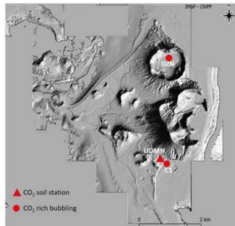
Figure 10 : Sites surveillés du réseau géochimique de Mayotte. Les variations du flux de CO 2 dans le sol sont étroitement liées aux processus magmatiques profonds qui peuvent avoir lieu au niveau du manteau (Liuzzo et al., 2021). La composition chimique et isotopique des bullages de gaz est potentiellement influencée par des processus se produisant dans le système hydrothermal crustal (©OVPF-IPGP / REVOSIMA).
