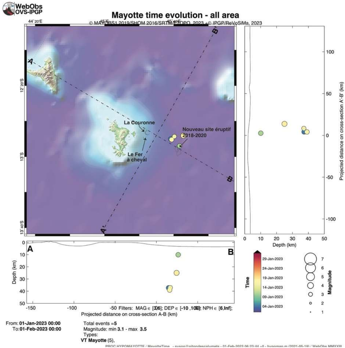
Figure 1c : Carte de localisation des épicentres ( \pm 5 km) des séismes volcano-tectoniques (VT) de magnitude M \geq 3 entre le 1 er et le 31 janvier 2023 enregistrés avec les réseaux sismiques à terre (IPGP-IFREMER-CNRS-BRGM-BCSF-RENASS, ITES). Sont aussi représentées une projection des hypocentres des séismes le long de coupes transverses et axiales le long de la ride montrant la localisation estimée en profondeur (la précision varie entre \pm 5 km et \pm 15 km) des séismes en fonction de la magnitude (taille des symboles) et de la date (échelle temporelle de couleur). Les structures volcaniques de la zone dite de « La Couronne », du « Fer à cheval » sont indiquées en grisé tout comme les coulées de lave de Fani Maoré. De nombreux points de sortie de panaches de fluides dans la colonne d'eau ont été identifiés dans la structure du Fer à Cheval avec une signature géochimique magmatique (voir section Géochimie des fluides). © OVPF-IPGP, BRGM, IFREMER, CNRS, BCSF-RENASS, ITES / REVOSIMA).
