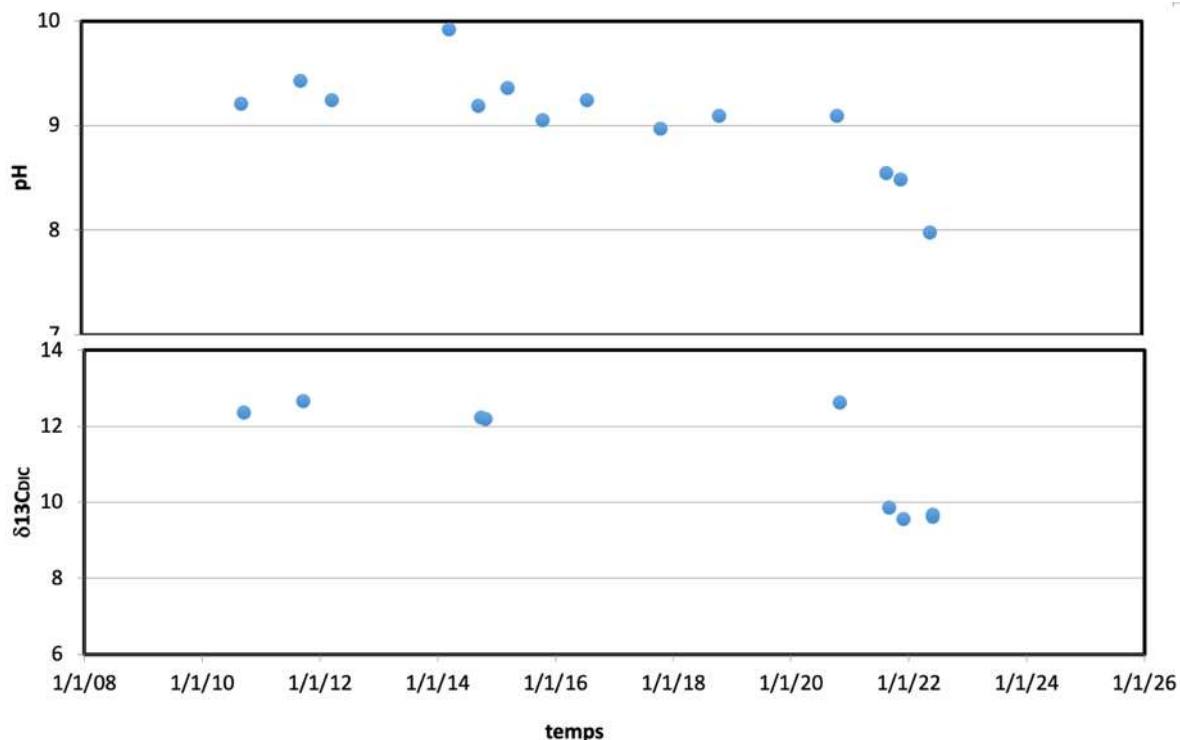
Figure 15 : Évolution temporelle du pH et du \delta^{13}\text{C}_{\text{DIC}} des eaux du Dziani Dzaha entre 2010 et 2022 (données antérieures à 2015 ( Sarazin et al., 2021 ; Cadeau et al., 2020 ), données de 2014 à 2021 incluses ( Cadeau et al., 2022 )).
