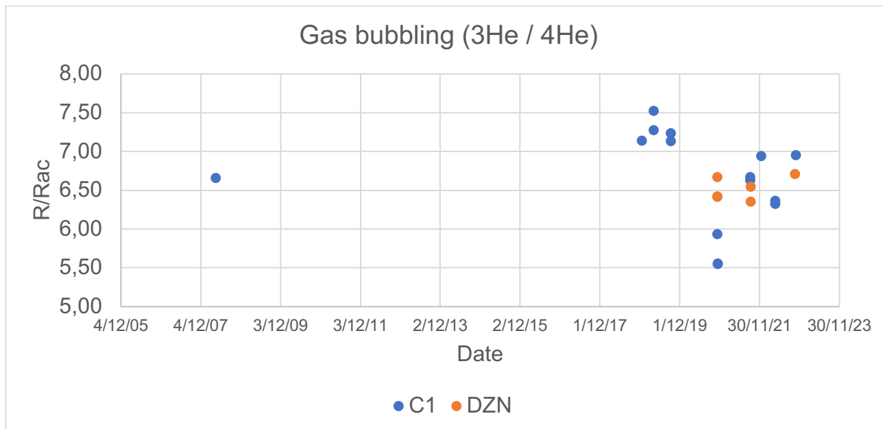
Figure 13 : Analyses isotopiques (gaz rares) des bullages au points de contrôle C1 (estran de l'aéroport) et DZN (Lac Dziani). Une augmentation du R/Ra (rapport isotopique de l'He normalisé à celui de l'atmosphère) est liée à une augmentation de la contribution des fluides profonds remontant du manteau. Erreur moyenne sur chaque analyse : 0.05 unité.
