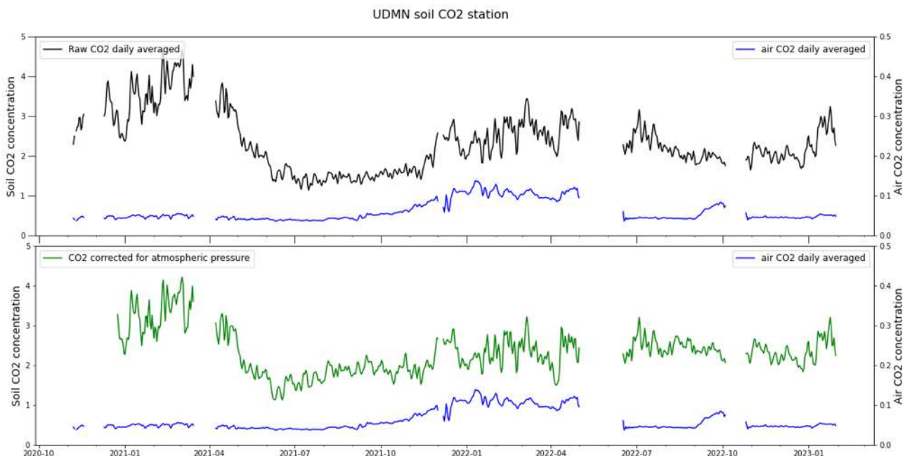
Figure 11 : Concentration en CO 2 dans le sol à la station permanente UDMN. Comparaison entre les données brutes (noir) et les données corrigées de l'influence de la pression atmosphérique (vert). Bleu : concentration dans l'air (1 m au-dessus du sol). Les variations de concentrations dans l'air sont liées à l'activité biogénique (©OVPF-IPGP / REVOSIMA).
