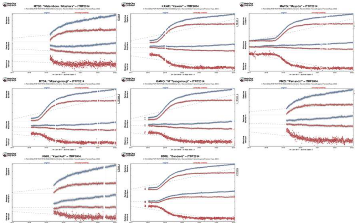
Figure 9 : Déplacements (en cm) enregistrés sur les 8 stations GPS localisés à Mayotte (MTSB, KAWL, MAYG, M TSA, GAMO, PMZI, KNKL, BDRL ; la station PORO a été retirée en 2021 et n'est donc plus affichée ici) entre le 1 er janvier 2017 et 31 janvier 2023 pour visualiser une longue série temporelle ante crise. En bleu les données brutes, en rouge les données corrigées du mouvement de la plaque. Les stations sont présentées dans un ordre géographique ; du nord au sud (de haut en base à et d'ouest en est (de gauche à droite). Post-traitement de ces données réalisé par l'IPGP (©OVPF-IPGP / REVOSIMA).
