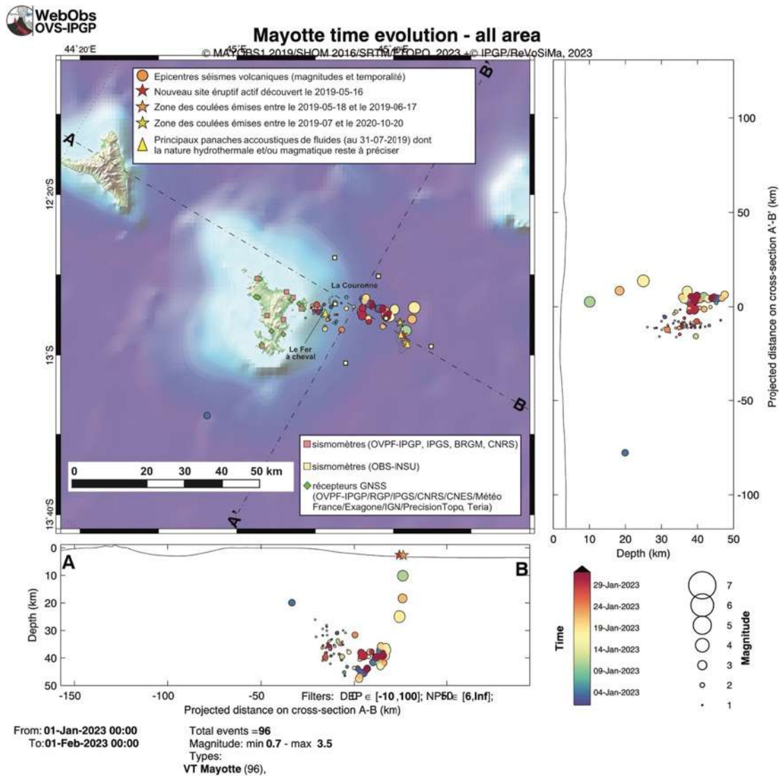
Figure 1a : Carte des épicentres ( \pm 5 km) des séismes volcano-tectoniques (VT) localisés avec les réseaux sismiques à terre (IPGP-CNRS-BRGM-BCSF-RENAISS, ITES) entre le 1 er et 31 janvier 2023 (échelle temporelle de couleur). Sont aussi représentées une projection des hypocentres des séismes le long de coupes transverses et axiales le long de la ride montrant la localisation estimée en profondeur (la précision varie entre \pm 5 km et \pm 15 km) des séismes en fonction de la magnitude (taille des symboles et de la date (échelle temporelle de couleur)). La localisation approximative des panaches acoustiques identifiés pendant les campagnes océanographiques (MD220-MAYOBS1, MD221-MAYOBS2, MD222-MAYOBS3, MD223-MAYOBS4, MAYOBS15, MAYOBS17) et dont la nature hydrothermale et/ou magmatique reste à préciser, est indiquée par des triangles jaunes, l'étoile rouge indique le site éruptif nouvellement identifié le 16 mai 2019, l'étoile orange la zone des coulées émises entre le 18/05/2019 et le 17/06/2019 et l'étoile jaune la zone des coulées émises entre juillet 2019 et le 18/01/2021. Les structures volcaniques de la zone dite de « La Couronne », du « Fer à cheval » sont indiquées en grisé tout comme les coulées de lave de Fani Maoré. Les stations sismiques du réseau terrestre, les sismomètres fond de mer (OBS) et les stations de positionnement par satellite GPS sont indiquées par des symboles (voir légende). (©OVPF-IPGP, BRGM, IFREMER, CNRS, BCSF-RENAISS, ITES / REVOSIMA).
