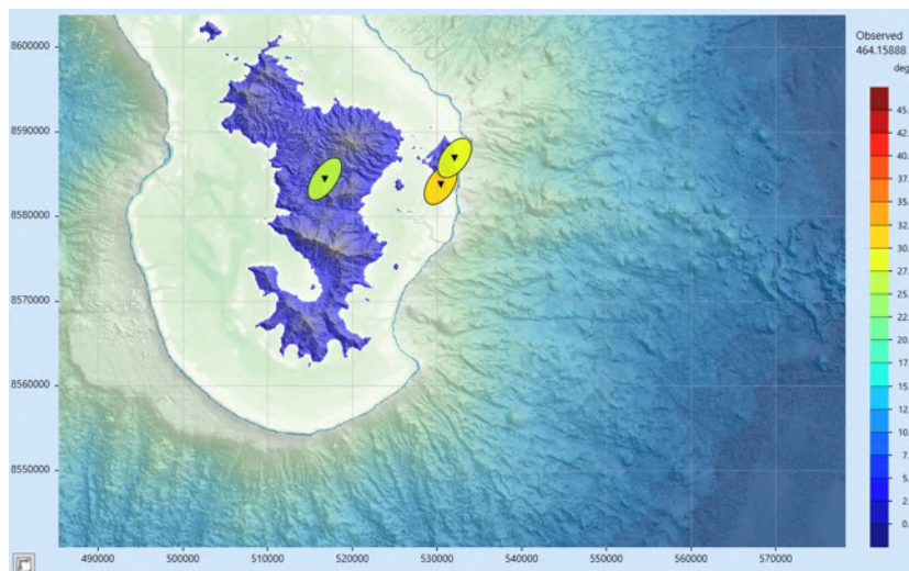
Figure 18 : Carte de tenseurs de phases calculés à 460 secondes des 3 stations MT pour le mois d'août 2023 (@BRGM et REVOSIMA).
