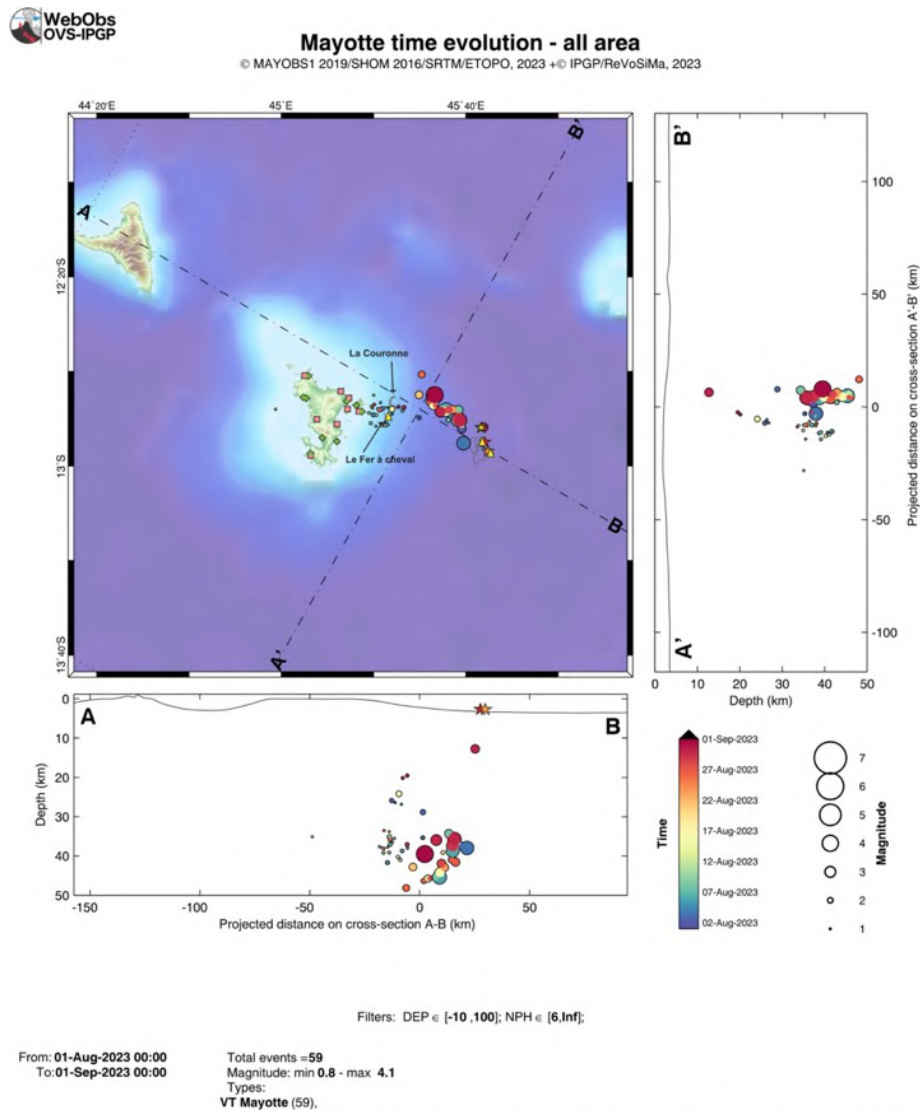
Figure 2 : Carte des épicentres ( \pm 5 km) des séismes volcano-tectoniques (VT) localisés avec les réseaux sismiques à terre (IPGP-CNRS-BRGM-BCSF-RENASS, ITES) entre le 1 er et 31 août 2023 (échelle temporelle de couleur). Sont aussi représentées une projection des hypocentres des séismes le long de coupes transverses et axiales le long de la ride montrant la localisation estimée en profondeur (la précision varie entre +5 km et +-15 km) des séismes en fonction de la magnitude (taille des symboles) et de la date (échelle temporelle de couleur). La localisation approximative des panaches acoustiques identifiés pendant les campagnes océanographiques (MD220-MAYOBS1, MD221-MAYOBS2, MD222-MAYOBS3, MD223-MAYOBS4, MAYOBS15, MAYOBS17 ; Rinnert et al., 2019) et dont la nature hydrothermale et/ou magmatique reste à préciser, est indiquée par des triangles jaunes, l'étoile rouge indique le site éruptif nouvellement identifié le 16 mai 2019, l'étoile orange la zone des coulées émises entre le 18/05/2019 et le 17/06/2019 et l'étoile jaune la zone des coulées émises entre juillet 2019 et le 18/01/2021. Les structures volcaniques de la zone dite de « La Couronne », du « Fer à cheval » sont indiquées en grisé tout comme les coulées de lave de Fani Maoré. Les stations sismiques du réseau terrestre et les stations de positionnement par satellite GPS sont indiquées par des symboles (voir légende). (©OVPF-IPGP, BRGM, IFREMER, CNRS, BCSF-RENASS, ITES / REVOSIMA).
