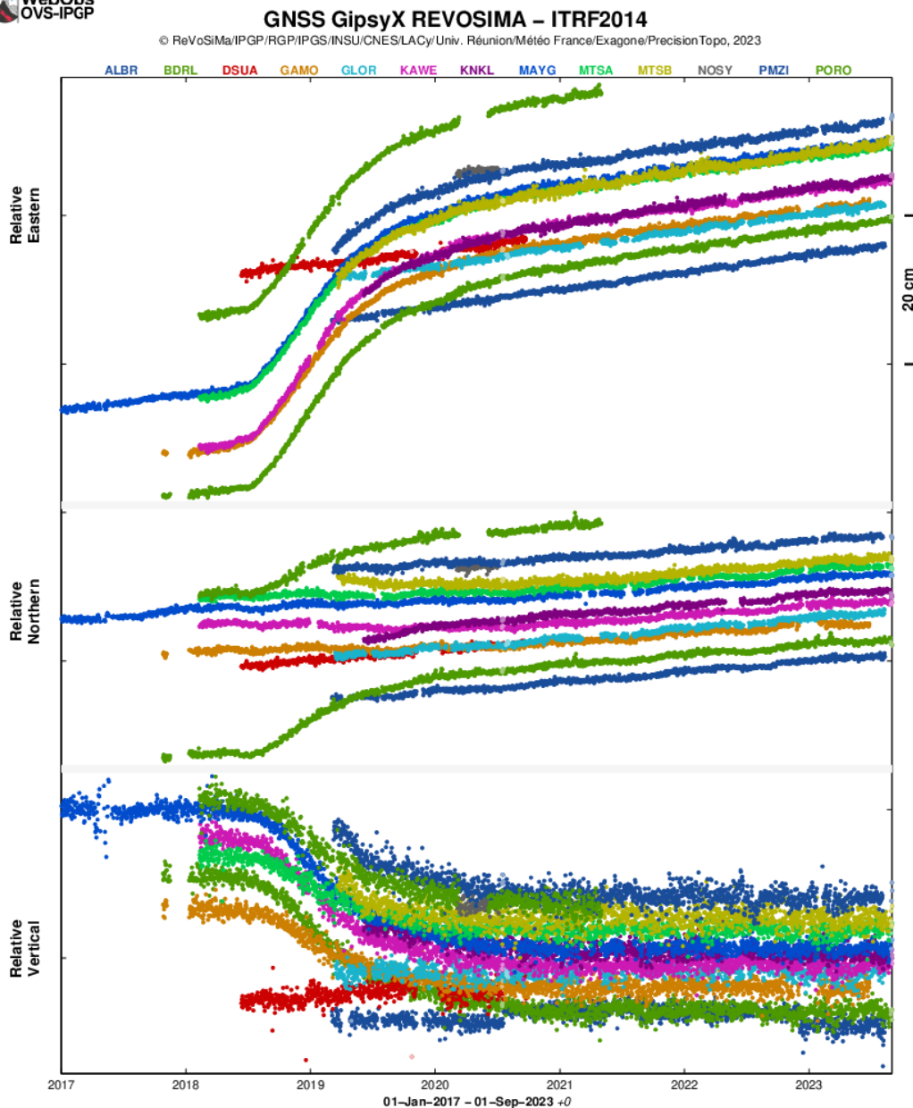
Figure 9 : Déplacements (en cm) enregistrés sur 9 stations GPS localisés à Mayotte (BDRL, GAMO, KAWA, KNKL, MAYG, MTSB, MTSB, PMZI, PORO), 1 station à Grande Glorieuse (GLOR), 1 station à Aldabra (ALBR) et 2 stations au nord de Madagascar à Diego Suarez (DSUA) et Nosy Be (NOSY) sur les composantes est (en haut), nord (au milieu) et vertical (en bas) entre le 1 er janvier 2017 et le 31 août 2023 pour visualiser une longue série temporelle ante crise. Post-traitement de ces données réalisé par l'IPGP (©OVPF-IPGP / REVOSIMA).
