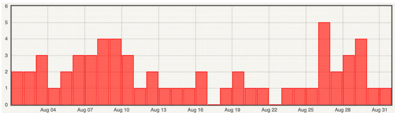
Figure 7 : Histogramme représentant le nombre de séismes par jour localisés en août 2023 par le réseau sismologique du REVOSIMA. En rouge les séismes volcano-tectoniques, en orange les séismes longues périodes, en jaune les séismes très longues périodes (© OVVPF-IPGP et REVOSIMA).
