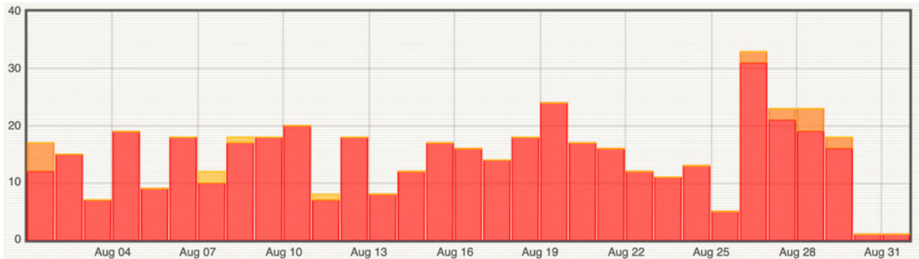
Figure 6 : Histogramme représentant le nombre de séismes par jour détectés en août 2023 par le réseau sismologique du REVOSIMA. En rouge les séismes volcano-tectoniques, en orange les séismes longues périodes, en jaune les séismes très longues périodes (© OVVPF-IPGP et REVOSIMA).
