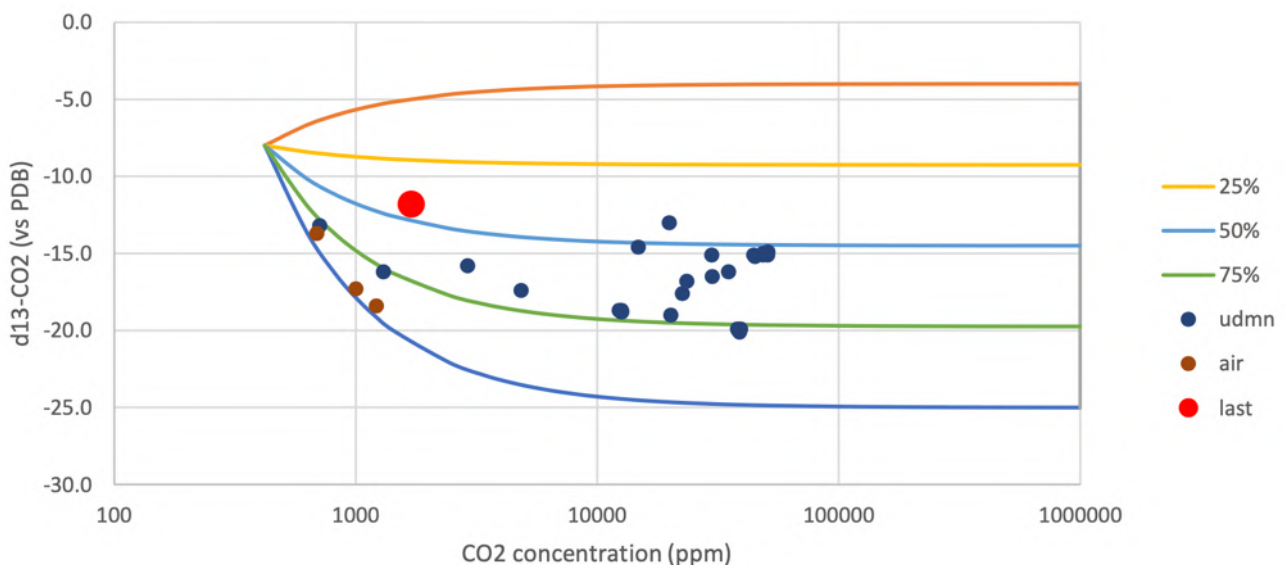
Figure 13 : Variations isotopiques du carbone ( \delta^{13}\text{C} -CO 2 ) du CO 2 dans l'air et dans les gaz du sol à la station UDMN. La composition du pôle magmatique est fixée à -4.0 per mil (signature des bullages du site C1 – estran de l'aéroport).
