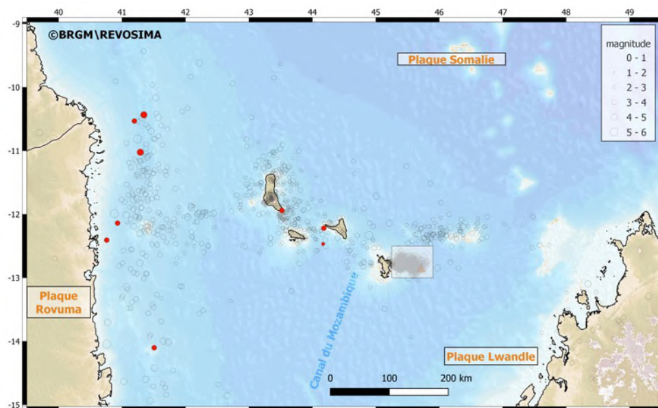
Figure 1: Sismicité régionale enregistrée depuis 2018 (modifié d'après Bertil et al. , 2021). Les séismes d'août 2023 sont représentés en rouge. Le fond de carte est construit à partir des données topographiques et bathymétriques de Gebco 2022 ( www.gebco.net ). Le trait de côte et les frontières administratives sont extraits de https://gadm.org/ . Le carré blanc encadre les essaims sismiques surveillés depuis 2018. Se référer aux Figures 2 et 3 de ce bulletin pour la distribution de cette sismicité.
