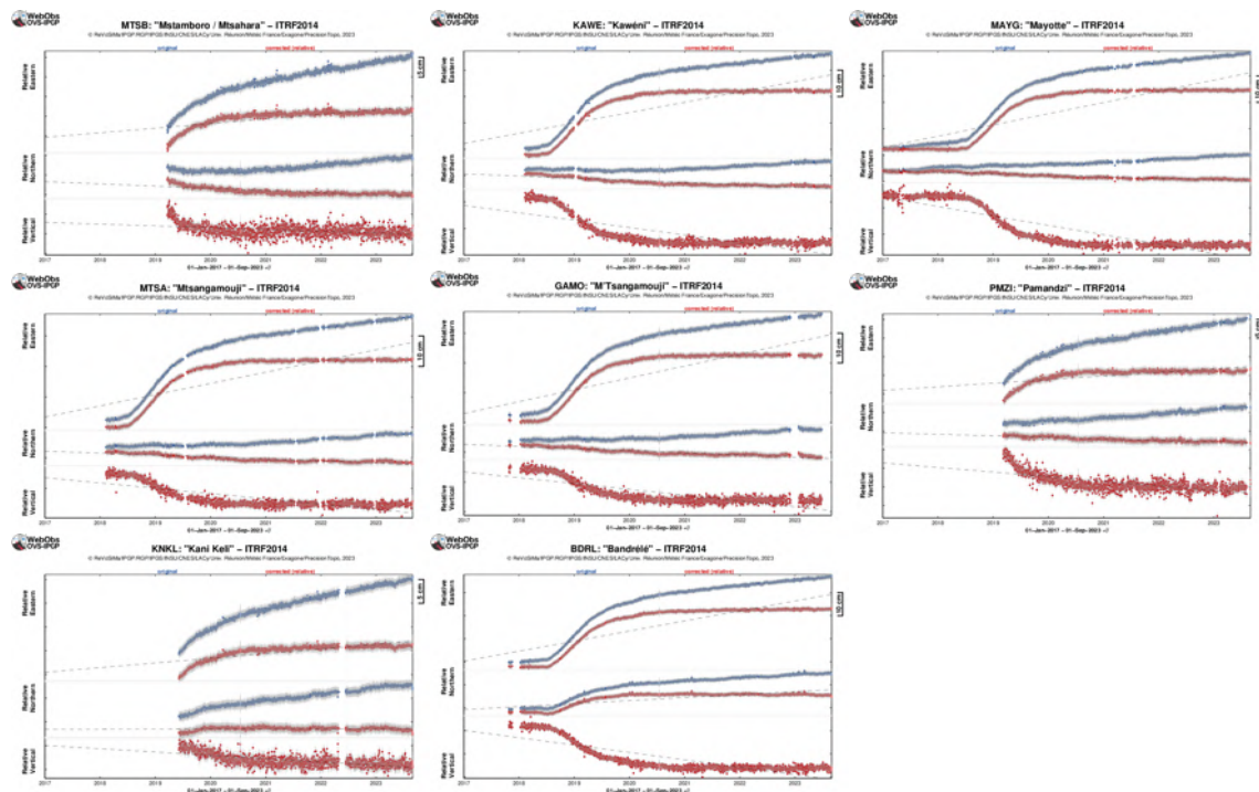
Figure 10 : Déplacements (en cm) enregistrés sur les 8 stations GPS localisés à Mayotte (MTSB, KAWI, MAYG, M TSA, GAMO, PMZI, KNKL, BDRL ; la station PORO a été retirée en 2021 et n'est donc plus affichée ici) entre le 1 er janvier 2017 et le 31 août 2023 pour visualiser une longue série temporelle ante crise. En bleu les données brutes, en rouge les données corrigées du mouvement de la plaque. Les stations sont présentées dans un ordre géographique ; du nord au sud (de haut en base à et d'ouest en est (de gauche à droite). Post-traitement de ces données réalisé par l'IPGP (©OVPF-IPGP / REVOSIMA).
