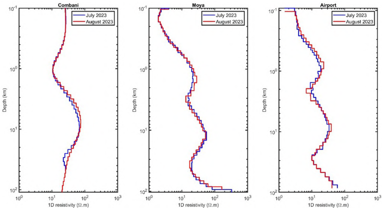
Figure 19 : Modèles 1D de résistivité du sous-sol de 100 m à 100 km de profondeur sous Combani (gauche), Moya (centre) et Aéroport (droite) pour les mois de Juillet (bleu) et Aout 2023 (rouge).
