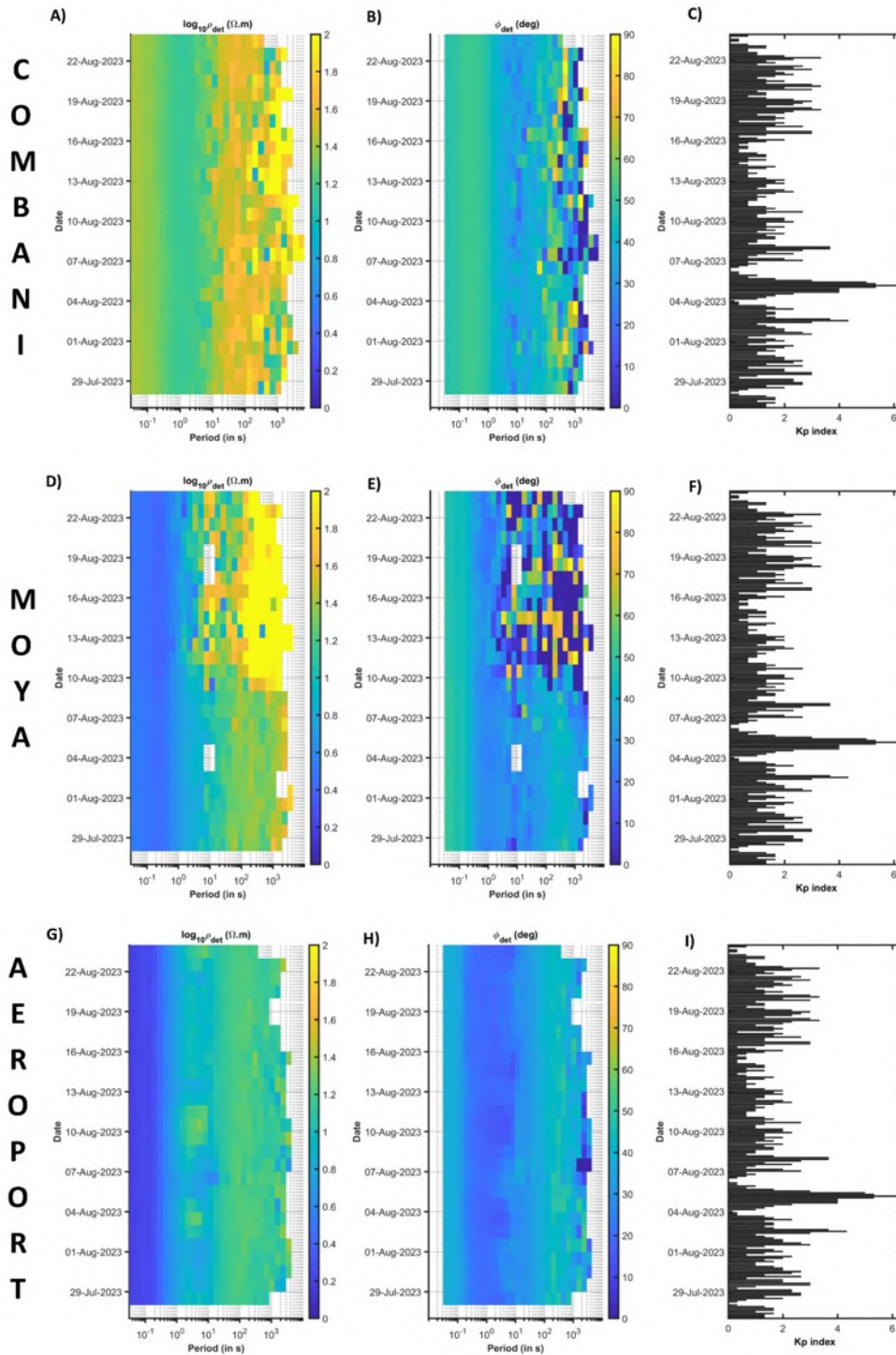
Figure 21 : Période du 26/07/2023 au 26/08/2023 - Chroniques temps-période de résistivité apparente de l'invariant 1D MT en échelle logarithmique (a, d, g), de phases (b, e, h) et index géomagnétiques Kp (c, f, i) du réseau MT Revosima (©BRGM et REVOSIMA) pour le site de Combani (haut), Moya (centre) et Aéroport (bas).
