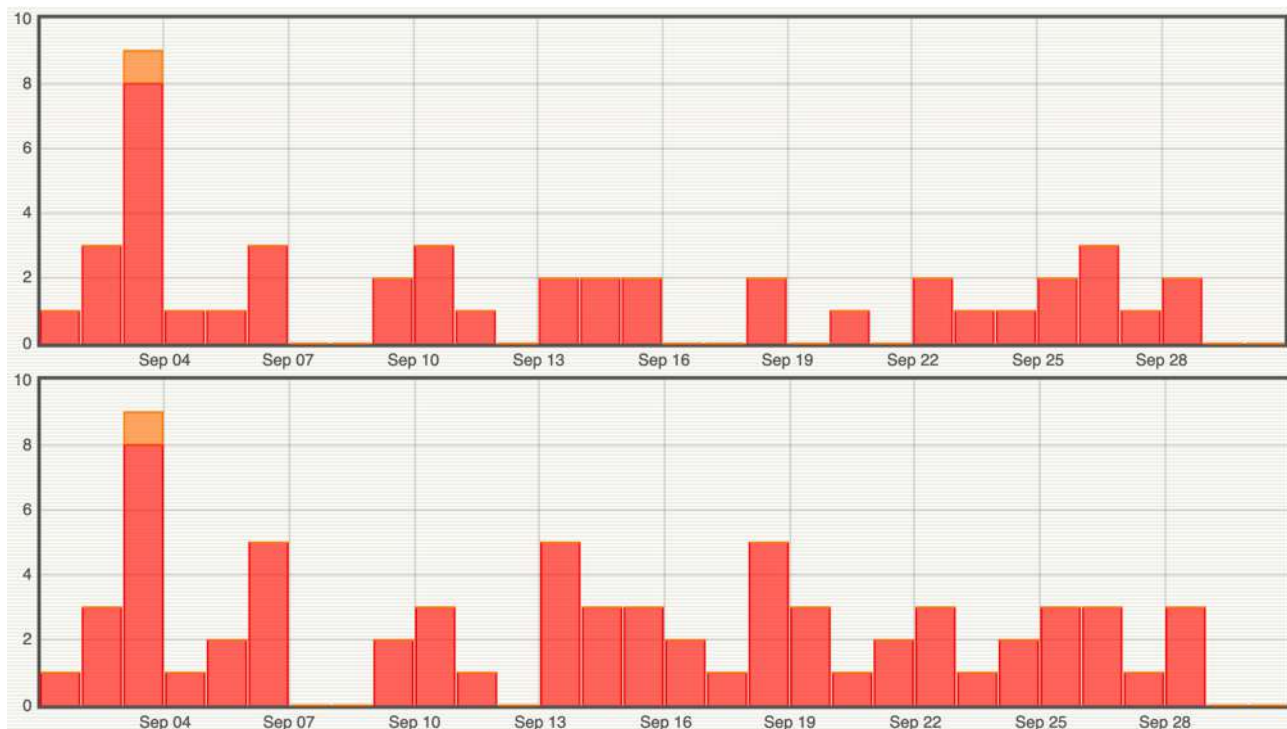
Figure 7 : Histogramme représentant le nombre de séismes par jour détectés (en haut) et localisés (en bas) en septembre 2023 par le réseau sismologique du REVOSIMA. En rouge les séismes volcano-tectoniques, en orange les séismes longues périodes, en jaune les séismes très longues périodes (© OVPF-IPGP et REVOSIMA).
