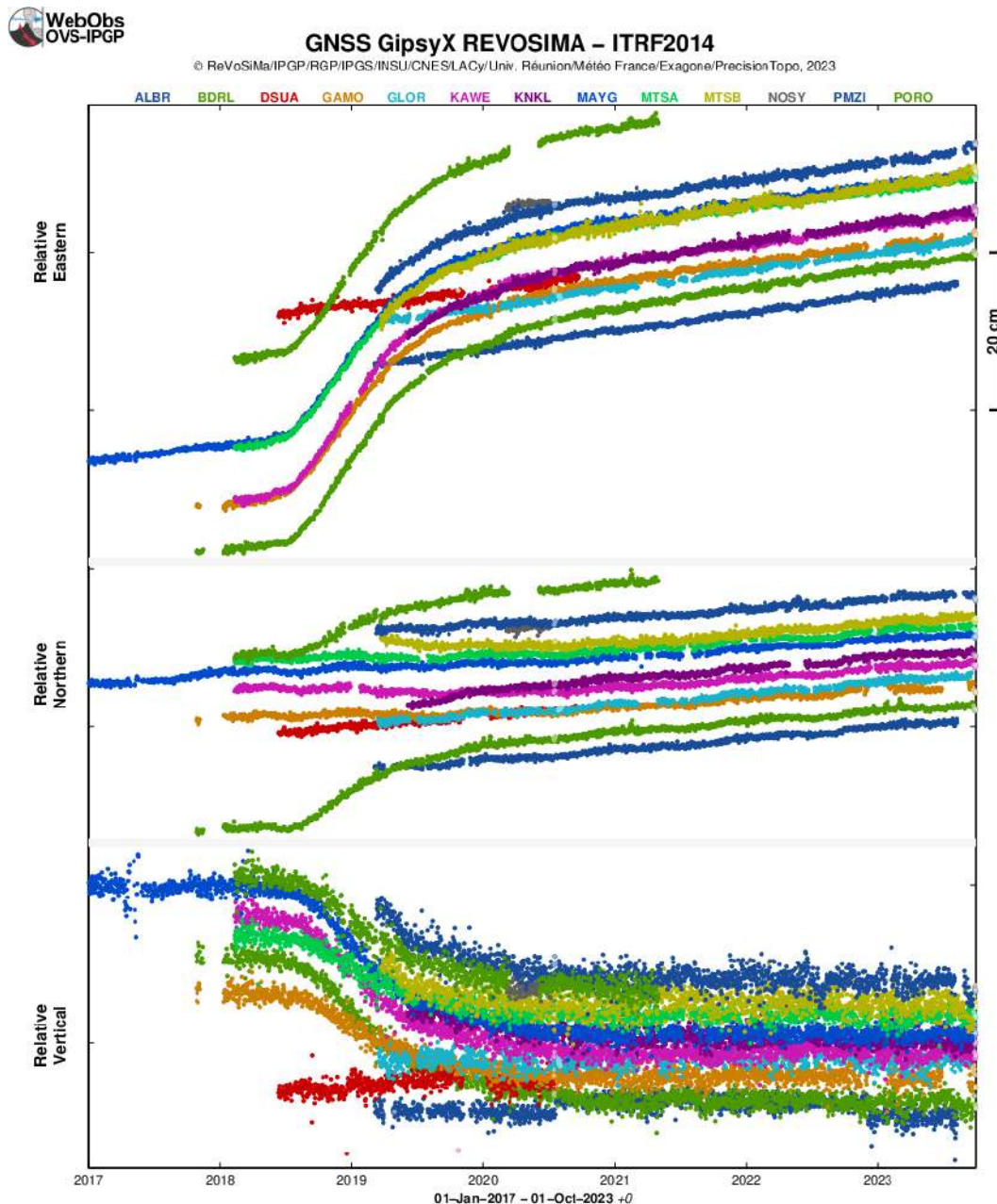
Figure 9 : Déplacements (en cm) enregistrés sur 9 stations GPS localisées à Mayotte (BDRL, GAMO, KAWE, KNKL, MAYG, MTSB, PMZI, PORO), 1 station à Grande Glorieuse (GLOR), 1 station à Aldabra (ALBR) et 2 stations au nord de Madagascar à Diego Suarez (DSUA) et Nosy Be (NOSY) sur les composantes est (en haut), nord (au milieu) et vertical (en bas) entre le 1 er janvier 2017 et le 30 septembre 2023 pour visualiser une longue série temporelle ante crise. Post-traitement de ces données réalisé par l'IPGP (©OVPF-IPGP / REVOSIMA).
