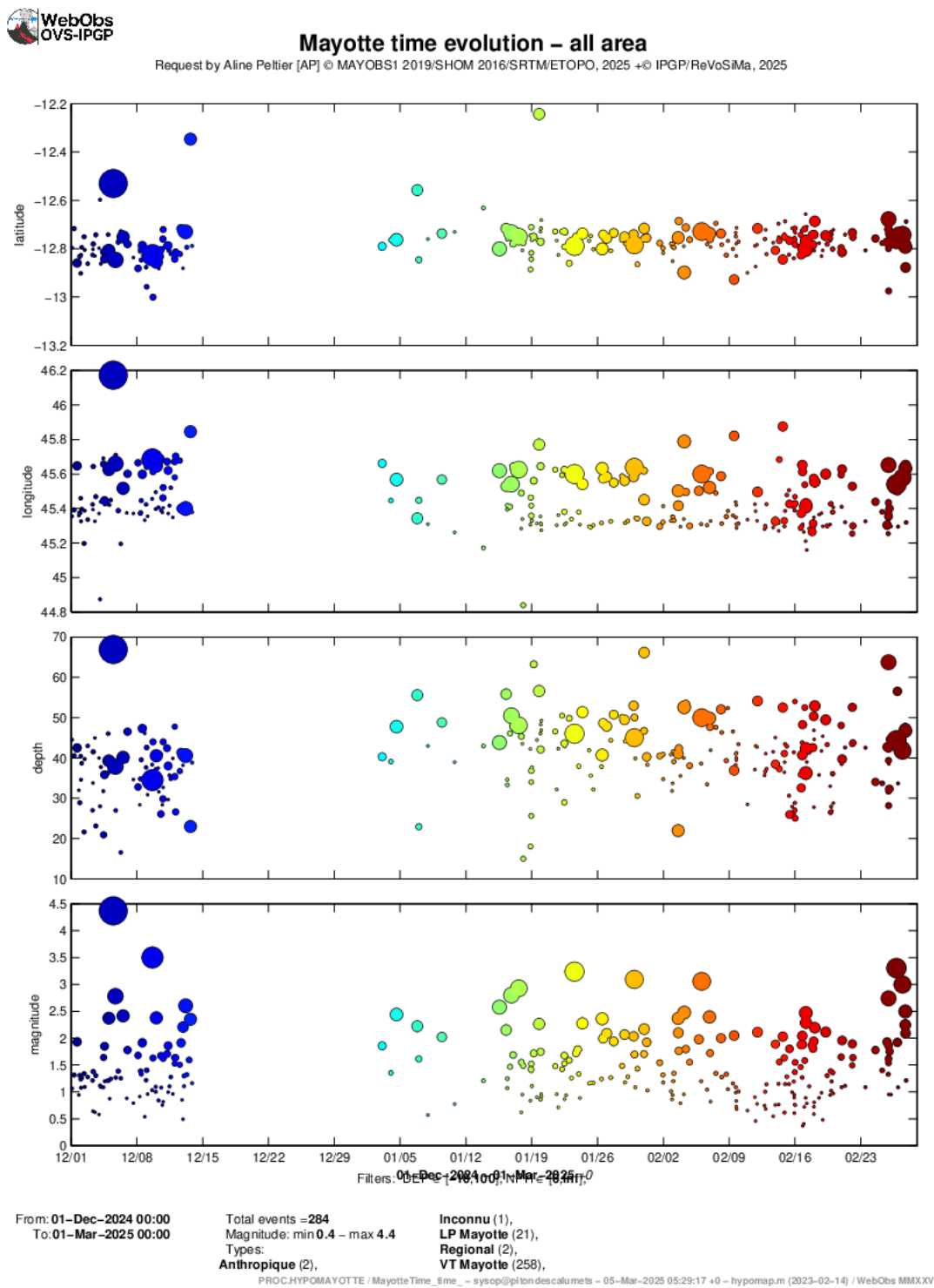
Figure 5 : Variation temporelle (échelle de couleur) des principaux paramètres (latitude, longitude, profondeur et magnitude) de la sismicité enregistrée et localisée par le REVOSIMA avec les réseaux sismiques à terre (IPGP-CNRS-BRGM-BCSF-RENASS, ITES) entre le 1 er décembre 2024 et le 28 février 2025 (3 mois) (© OVPF- IPGP, BRGM, IFREMER, CNRS, BCSF-RENASS, ITES / REVOSIMA). A noter que le séisme de magnitude 4.5 correspond au séisme régional ressenti du 5 décembre 2024.
