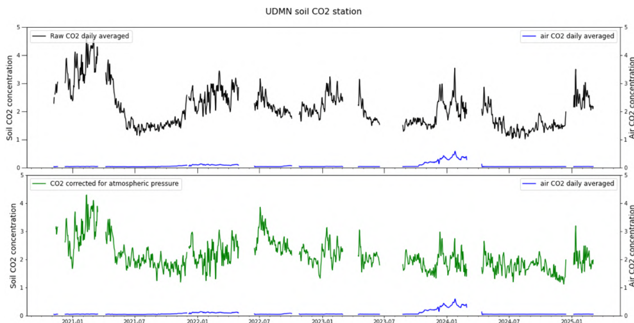
Figure 12 : Concentration en \text{CO}_2 dans le sol à la station permanente UDMN. Comparaison entre les données brutes (noir) et les données corrigées de l'influence de la pression atmosphérique (vert). Bleu : concentration du \text{CO}_2 dans l'air (1 m au-dessus du sol). Les variations de concentrations dans l'air sont liées à l'activité biogénique (©OVPF-IPGP / REVOSIMA).
