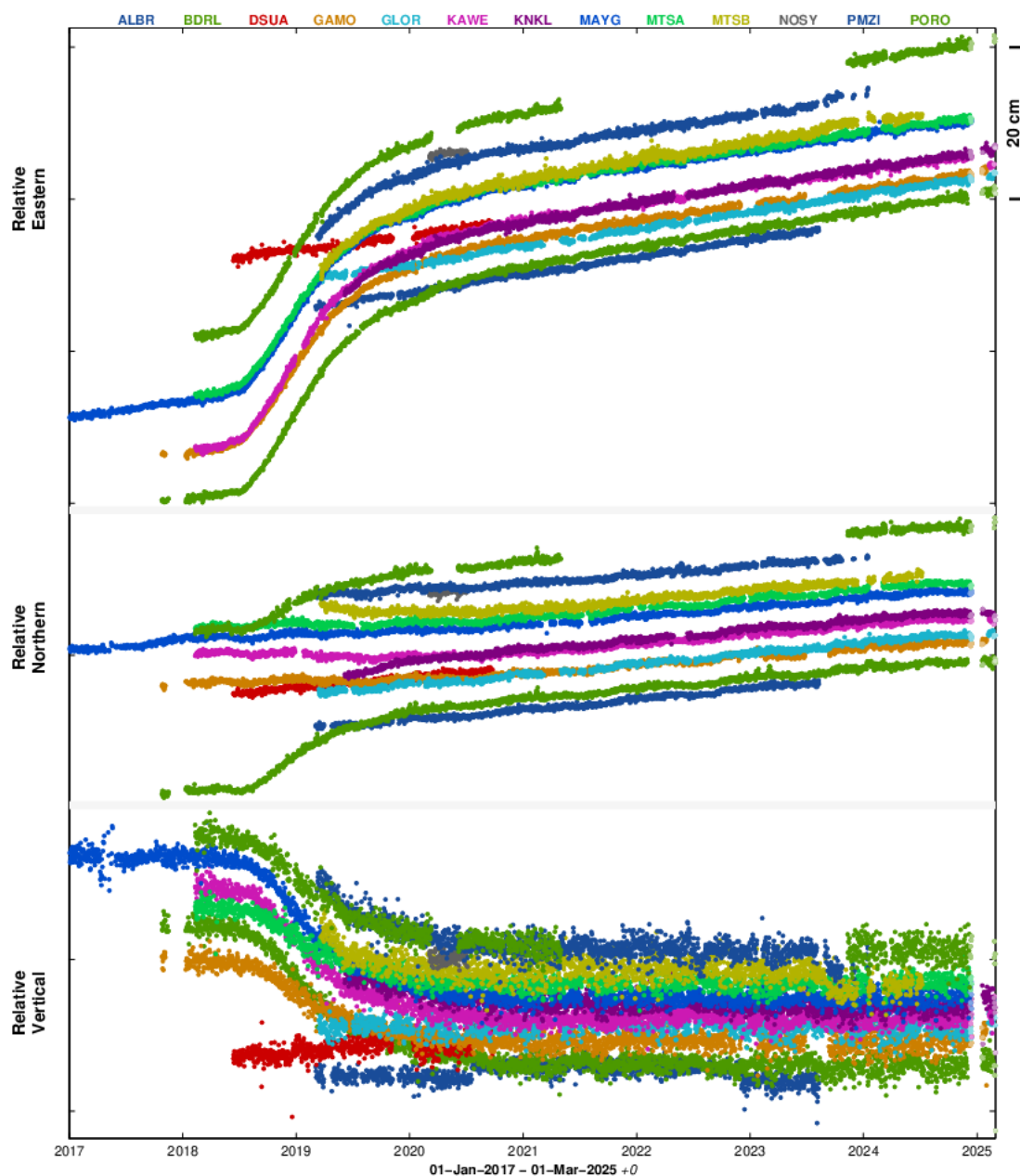
Figure 9 : Déplacements (en cm) enregistrés sur 9 stations GPS localisés à Mayotte (BDRL, GAMO, KAWA, KNKL, MAYG, MTSA, MTSB, PMZI, PORO), 1 station à Grande Glorieuse (GLOR), 1 station à Aldabra (ALBR) et 2 stations au nord de Madagascar à Diego Suarez (DSUA) et Nosy Be (NOSY) sur les composantes est (en haut), nord (au milieu) et vertical (en bas) entre le 1 er janvier 2017 et 28 février 2025 pour visualiser une longue série temporelle ante crise. Post-traitement de ces données réalisé par l'IPGP (©OVPF-IPGP / REVOSIMA). Suite au passage du cyclone Chido sur Mayotte le 14 décembre 2024, deux stations (MAYG et MTSA) ont été détruites, alors que les stations KNKL, KAWA, PORO, GAMO et BDRL ont subi des coupures électriques et/ou de transmission. Au retour des données, aucun changement de tendance n'a été observé.
