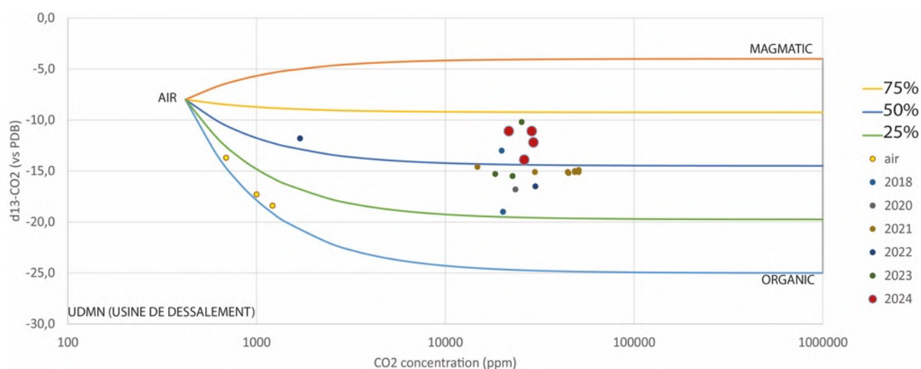
Figure 13 : Variations isotopiques du carbone ( \delta^{13}\text{C}-\text{CO}_2 ) du \text{CO}_2 dans l'air et dans les gaz du sol à la station UDMN. La composition du pôle magmatique est fixée à -4.0 per mil (signature des bullages du site C1 – estran de l'aéroport).
