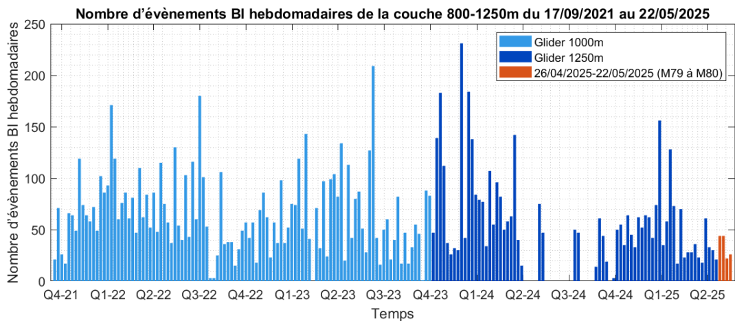
Figure 19 : Histogramme du nombre hebdomadaire de détections d'évènement BI (Backscatter Index) depuis le début de la surveillance par planeur (17/09/2021) et jusqu'au 22/05/2025 (fin de la mission 80). Résultats obtenus avec les planeurs limités à 1000 m d'immersion en bleu clair et à 1250 m d'immersion en bleu foncé. En orange, résultats pour la période entre le 26/04/2025 et le 22/05/2025 (Missions 79 et 80) avec le planeur limité à 1250 m d'immersion. L'échelle de temps est représentée par quartiles des années 2021 à 2025. Les périodes où le planeur n'a pas été utilisé sont symbolisées par un nombre d'évènements BI hebdomadaire égal à zéro.
