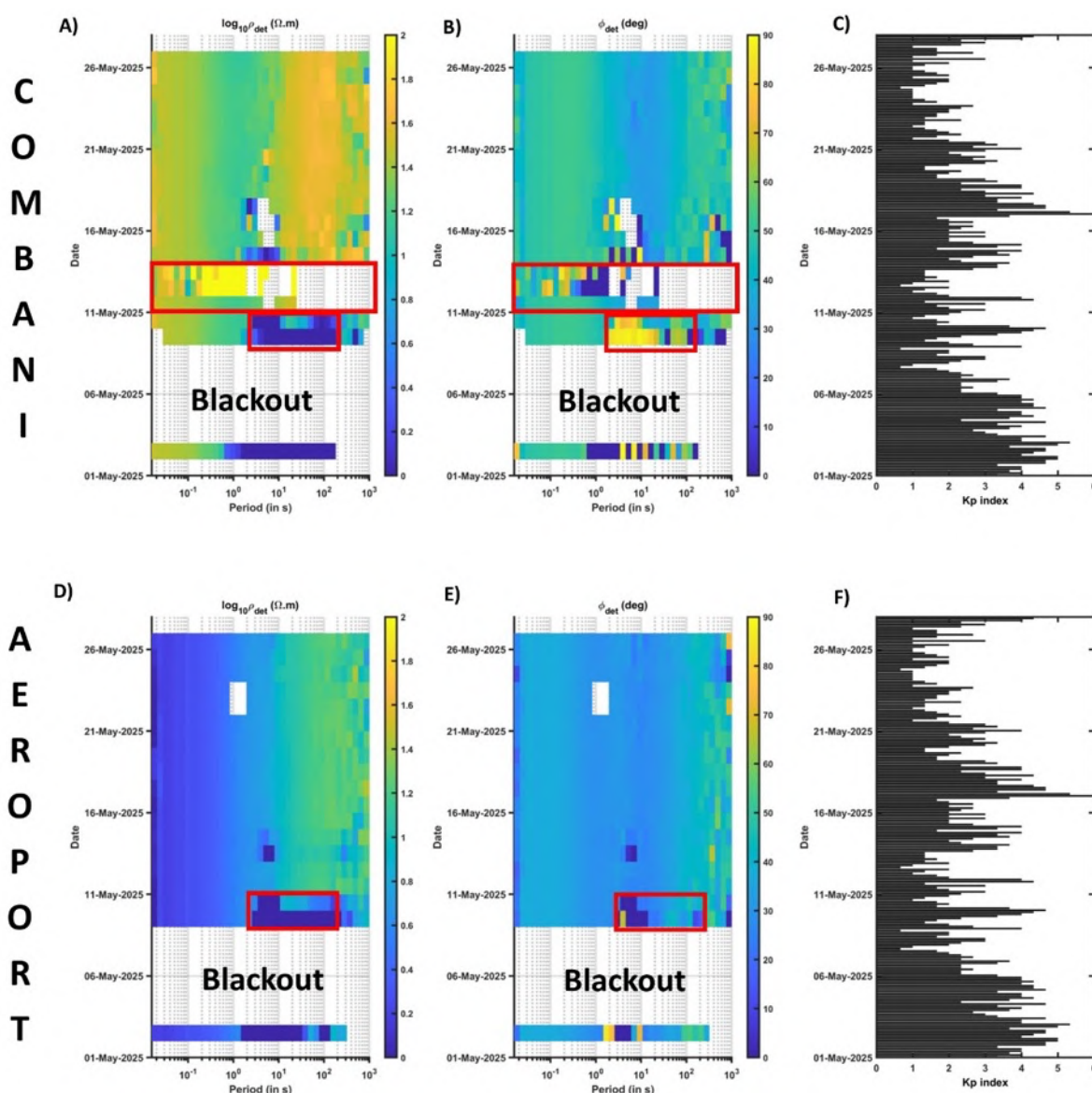
Figure 24 : Période du 01/05/2025 au 28/05/2025 - Chroniques temps-période de résistivité apparente de l'invariant 1D MT en échelle logarithmique (a, d), de phases (b, e) et l'index géomagnétique Kp (c, f) du réseau MT Revosima (©BRGM et REVOSIMA) pour le site de Combani (haut) et Aéroport (bas). Les carrés rouges mettent en évidence l'impact de bruits anthropiques sur les séries temporelles. On peut observer que l'orage géomagnétique du 17 mai permet d'obtenir courbes plus lisses en fréquences.
