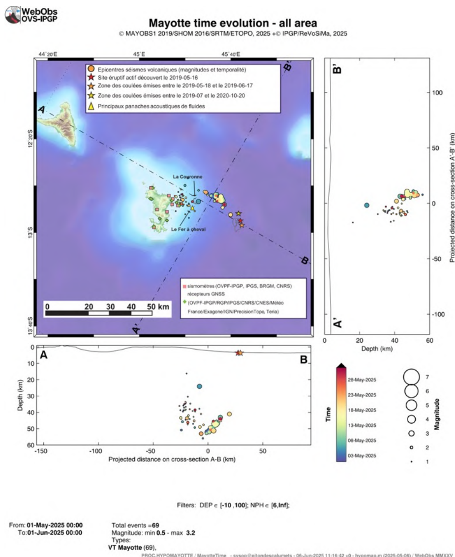
Figure 2 : Carte des épicentres ( \pm 5 km) des séismes volcano-tectoniques (VT) localisés avec les réseaux sismiques à terre (IPGP-CNRS-BRGM-BCSF-RENASS-ITES) en mai 2025 (échelle temporelle de couleur). Sont aussi représentées les projections des hypocentres des séismes le long de coupes transverses et axiales le long de la ride montrant la localisation estimée en profondeur (la précision varie entre \pm 5 km et \pm 15 km) des séismes en fonction de la magnitude (taille des symboles) et de la date (échelle temporelle de couleur). La localisation approximative des panaches acoustiques identifiés pendant les campagnes océanographiques est indiquée par des triangles jaunes, l'étoile rouge indique le site éruptif identifié le 16 mai 2019, l'étoile orange la zone des coulées émises entre le 18/05/2019 et le 17/06/2019 et l'étoile jaune la zone des coulées émises entre juillet 2019 et le 04/12/2020. Les structures volcaniques de la zone dites de « La Couronne » et du « Fer à Cheval » sont indiquées en grisé tout comme les coulées de lave de Fani Maoré. Les stations sismiques du réseau terrestre et les stations de positionnement par satellite GPS sont indiquées par des symboles (voir légende) (©OVPF-IPGP, BRGM, IFREMER, CNRS, BCSF-RENASS, ITES / REVOSIMA).
