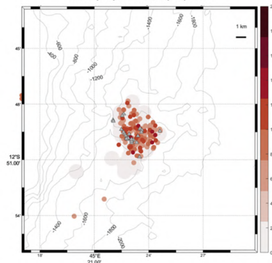
Anomalies de CO 2 (en \mu\text{mol/L} ) de la couche 800-1250m du 26/04/2025 au 22/05/2025
