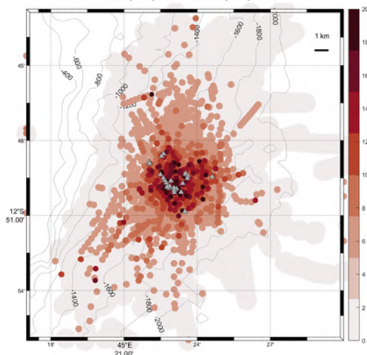
Anomalies de CO 2 (en \mu\text{mol/L} ) de la couche 0-1250m du 17/09/2021 au 22/05/2025
