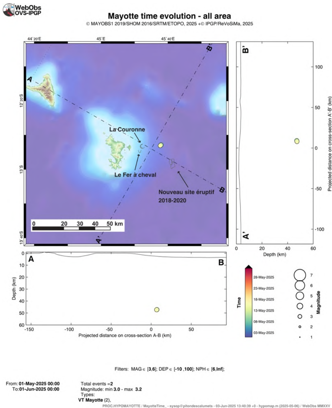
Figure 4 : Carte de localisation des épicentres ( \pm 5 km) des séismes de magnitude M \geq 3 en mai 2025 enregistrés avec les réseaux sismiques à terre (IPGP-IFREMER-CNRS-BRGM-BCSF-RENASS-ITES). Sont aussi représentées les projections des hypocentres des séismes le long de coupes transverses et axiales le long de la ride montrant la localisation estimée en profondeur (la précision varie entre \pm 5 km et \pm 15 km) des séismes en fonction de la magnitude (taille des symboles) et de la date (échelle temporelle de couleur). La localisation approximative des panaches acoustiques identifiés pendant les campagnes océanographiques est indiquée par des triangles jaunes, l'étoile rouge indique le site éruptif identifié le 16 mai 2019, l'étoile orange la zone des coulées émises entre le 18/05/2019 et le 17/06/2019 et l'étoile jaune la zone des coulées émises entre juillet 2019 et le 04/12/2020. Les structures volcaniques de la zone dites de « La Couronne » et du « Fer à Cheval » sont indiquées en grisé tout comme les coulées de lave de Fani Maoré (©OVPF-IPGP, BRGM, IFREMER, CNRS, BCSF-RENASS, ITES / REVOSIMA).
