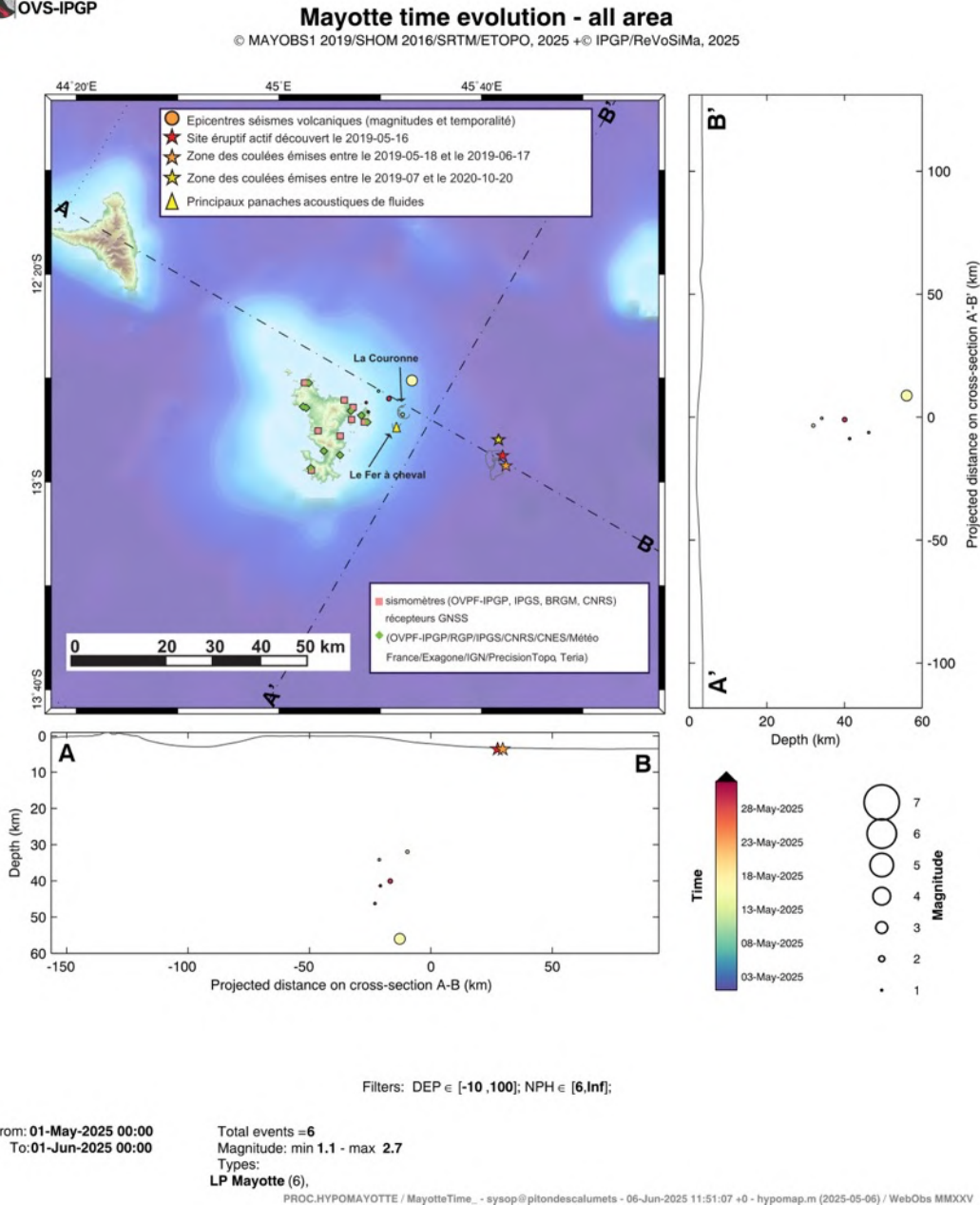
Figure 3 : Carte des épicentres ( \pm 5 km) des séismes longue période (LP) localisés avec les réseaux sismiques à terre (IPGP-CNRS-BRGM-BCSF-RENASS-ITES) en mai 2025 (échelle temporelle de couleur). Sont aussi représentées les projections des hypocentres des séismes le long de coupes transverses et axiales le long de la ride montrant la localisation estimée en profondeur (la précision varie entre \pm 5 km et \pm 15 km) des séismes en fonction de la magnitude (taille des symboles) et de la date (échelle temporelle de couleur). La localisation approximative des panaches acoustiques identifiés pendant les campagnes océanographiques est indiquée par des triangles jaunes, l'étoile rouge indique le site éruptif identifié le 16 mai 2019, l'étoile orange la zone des coulées émises entre le 18/05/2019 et le 17/06/2019 et l'étoile jaune la zone des coulées émises entre juillet 2019 et le 04/12/2020. Les structures volcaniques de la zone dites de « La Couronne » et du « Fer à Cheval » sont indiquées en grisé tout comme les coulées de lave de Fani Maoré. Les stations sismiques du réseau terrestre et les stations de positionnement par satellite GPS sont indiquées par des symboles (voir légende) (©OVPF-IPGP, BRGM, IFREMER, CNRS, BCSF-RENASS, ITES / REVOSIMA).
