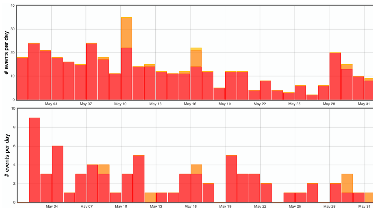
Figure 7 : Histogramme représentant le nombre de séismes par jour détectés (en haut) et localisés (en bas) en mai 2025 par le réseau sismologique du REVOSIMA. En rouge les séismes volcano-tectoniques, en orange les séismes longues périodes, en jaune les séismes très longues périodes (© OVPF-IPGP et REVOSIMA).
