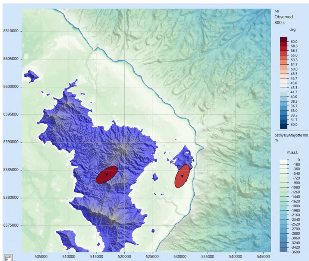
Figure 22 : Carte de tenseurs de phases calculés à 800 secondes des 2 stations MT actives du Revosima pour le mois de Mai 2025 (©BRGM et REVOSIMA). Les ellipses de tenseurs de phases sont colorées avec les valeurs de phase maximum \varphi_{\max} (en degrés) qui sont supérieures à 45°, traduisant ainsi une décroissance de résistivité en profondeur.
