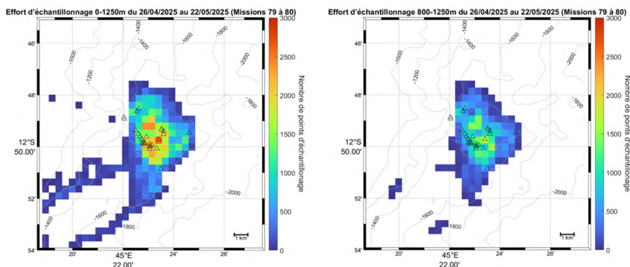
Figure 18 : Cartes centrées sur le Fer à Cheval représentant l'effort d'échantillonnage du planeur pour la période du 26/04/2025 au 22/05/2025 (missions 79 et 80) entre 0 et 1250 m de profondeur (à gauche), et entre 800 et 1250 m de profondeur (à droite). Le maillage est illustré par des cellules carrées mesurant 500 m de côté (0,25 km 2 ). La couleur représente le nombre de points d'échantillonnage réalisés dans chaque cellule. La bathymétrie est indiquée par des isobathes tous les 200 m. Les triangles noirs correspondent à la position du barycentre des sites actifs d'émissions de fluides déjà répertoriés (Scalabrin, C. (2023), https://doi.org/10.12770/070818f6-6520-49e4-bafd-9d4d0609bf7d ).
