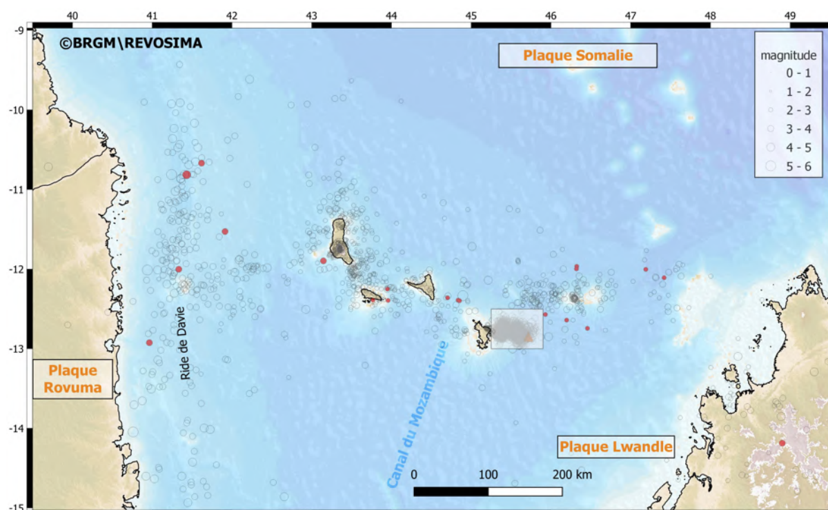
Figure 1: Sismicité régionale enregistrée depuis 2018 (modifié d'après Bertil et al., 2021). Les séismes de mai 2025 sont représentés en rouge. Le fond de carte est construit à partir des données topographiques et bathymétriques de Gebco 2022 ( www.gebco.net ). Le trait de côte et les frontières administratives sont extraits de https://gadm.org/ . Le carré blanc encadre les essaims sismiques surveillés depuis 2018. Se référer aux Figures 2 et 3 de ce bulletin pour la distribution de cette sismicité.
