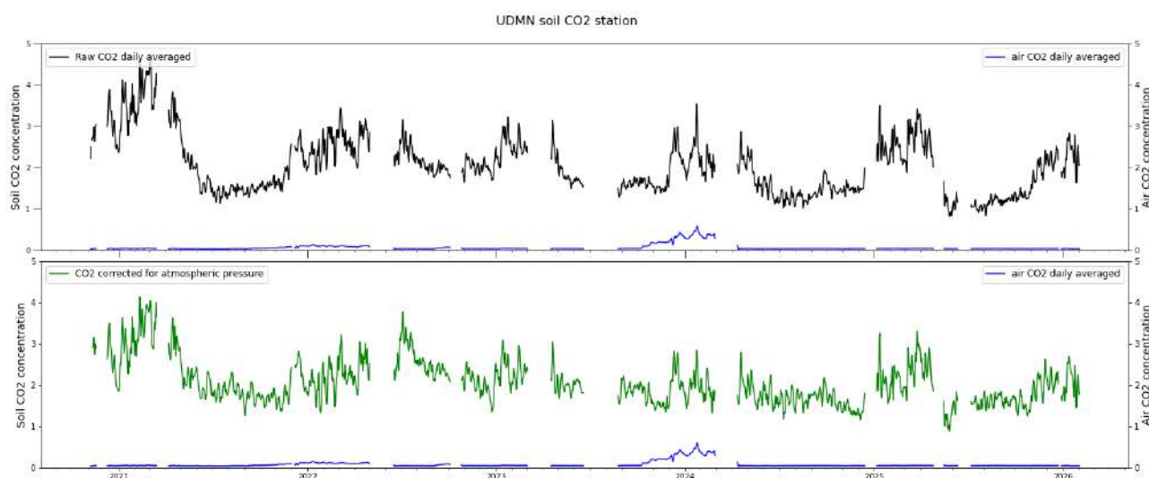
Figure 12 : Concentration en \text{CO}_2 dans le sol à la station permanente UDMN. Comparaison entre les données brutes (noir) et les données corrigées de l'influence de la pression atmosphérique (vert). Bleu : concentration du \text{CO}_2 dans l'air (1 m au-dessus du sol). Les variations de concentrations dans l'air sont liées à l'activité biogénique (©OVPF-IPGP / REVOSIMA).
