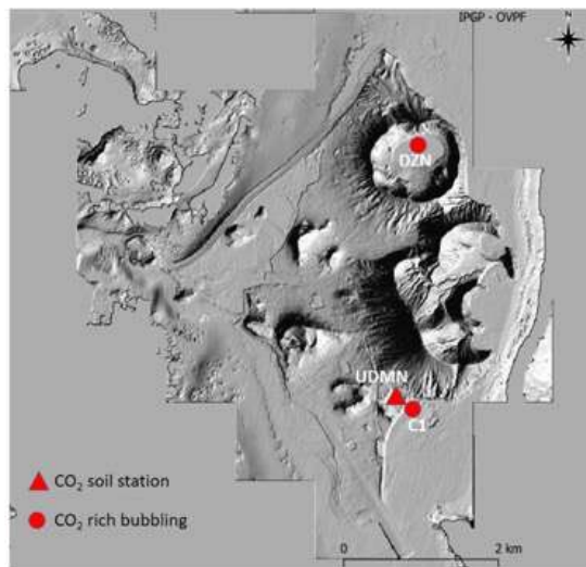
Figure 11 : Sites surveillés du réseau géochimique de Mayotte. Les variations du flux de \text{CO}_2 dans le sol sont étroitement liées aux processus magmatiques profonds qui peuvent avoir lieu au niveau du manteau (Di Muro et al. , 2016 ; Liuzzo et al. , 2021). La composition chimique et isotopique des bullages de gaz est potentiellement influencée par des processus se produisant dans le système hydrothermal crustal (©OVPF-IPGP / REVOSIMA).
