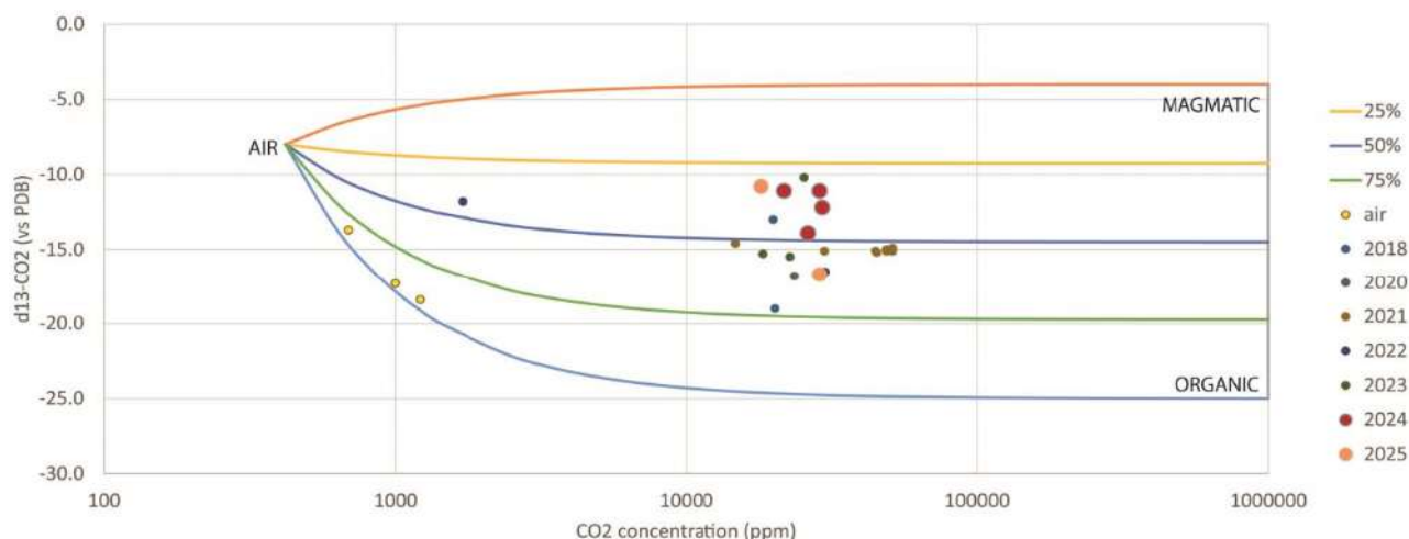
Figure 13 : Variations isotopiques du carbone ( \delta^{13}\text{C}-\text{CO}_2 ) du \text{CO}_2 dans l'air et dans les gaz du sol à la station UDMN. La composition du pôle magmatique est fixée à -4.0 per mil (signature des bullages du site C1 – estran de l'aéroport).
