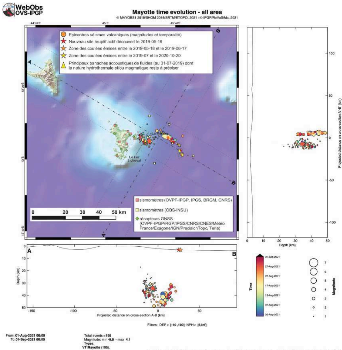
Figure 1a : Carte des épicentres (± 5 km) des séismes volcano-tectoniques (VT) localisés avec les réseaux sismiques à terre (IPGP-IFREMER-CNRS-BRGM-BCSF-RENASS, IPGS) entre le 1 er et 31 août 2021 (échelle temporelle de couleur). Sont aussi représentées une projection des hypocentres des séismes le long de coupes transverses et axiales le long de la ride montrant la localisation estimée en profondeur (la précision varie entre +5 km et -15 km) des séismes en fonction de la magnitude (taille des symboles et de la date (échelle temporelle de couleur)). La localisation approximative des panaches acoustiques identifiés pendant les campagnes océanographiques (MD220-MAYOBS1, MD221-MAYOBS2, MD222-MAYOBS3, MD223-MAYOBS4, MAYOBS15, MAYOBS17) et dont la nature hydrothermale et/ou magmatique reste à préciser, est indiquée par des triangles jaunes, l'étoile rouge indique le site éruptif nouvellement identifié le 16 mai 2019, l'étoile orange la zone des coulées émises entre le 18/05/2019 et le 17/06/2019 et l'étoile jaune la zone des coulées émises entre juillet 2019 et le 18/01/2021. Les structures volcaniques de la zone dite de « La Molaire » sont indiquées en grisé tout comme les coulées de lave du site éruptif. Les stations sismiques du réseau terrestre, les sismomètres fond de mer (OBS) et les stations de positionnement par satellite GPS sont indiquées par des symboles (voir légende). (©OVPF-IPGP, BRGM, IFREMER, CNRS, BCSF-RENASS, IPGS / REVOSIMA).
