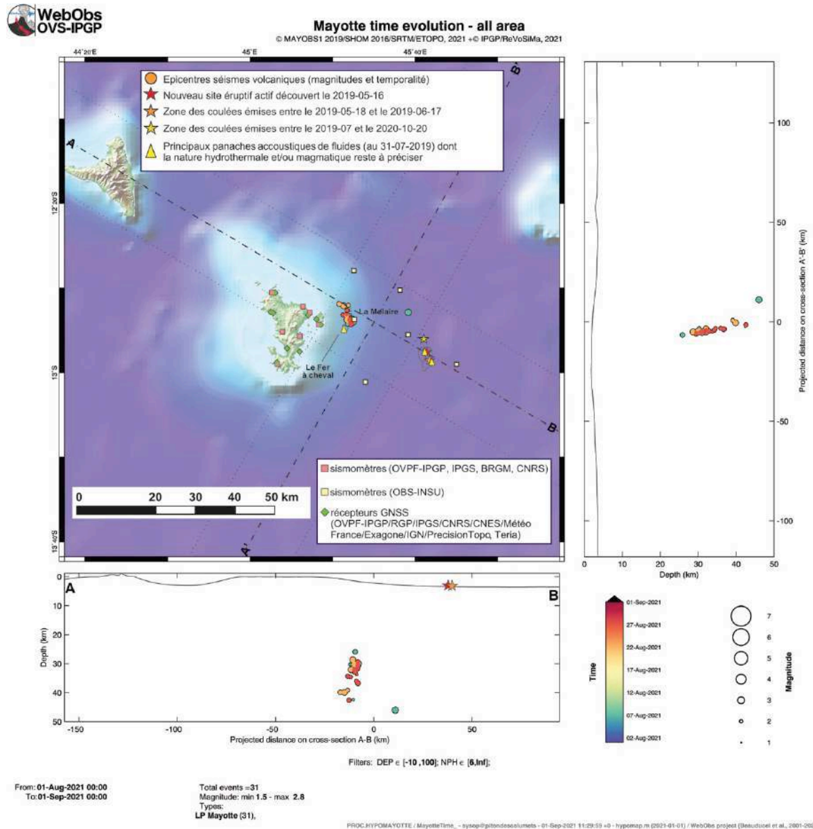
Figure 1b : Carte des épicentres ( \pm 5 km) des séismes longue période (LP) localisés avec les réseaux sismiques à terre (IPGP-IFREMER-CNRS-BRGM-BCSF-RENASS, IPGS) entre le 1 er et 31 août 2021 (échelle temporelle de couleur). Sont aussi représentées une projection des hypocentres des séismes le long de coupes transverses et axiales le long de la ride montrant la localisation estimée en profondeur (la précision varie entre \pm 5 km et \pm 15 km) des séismes en fonction de la magnitude (taille des symboles et de la date (échelle temporelle de couleur)). La localisation approximative des panaches acoustiques identifiés pendant les campagnes océanographiques (MD220-MAYOBS1, MD221-MAYOBS2, MD222-MAYOBS3, MD223-MAYOBS4, MAYOBS15, MAYOBS17) et dont la nature hydrothermale et/ou magmatique reste à préciser, est indiquée par des triangles jaunes, l'étoile rouge indique le site éruptif nouvellement identifié le 16 mai 2019, l'étoile orange la zone des coulées émises entre le 18/05/2019 et le 17/06/2019 et l'étoile jaune la zone des coulées émises entre juillet 2019 et le 18/01/2021. Les structures volcaniques de la zone dite de « La Molaire » sont indiquées en grisé tout comme les coulées de lave du site éruptif. Les stations sismiques du réseau terrestre, les sismomètres fond de mer (OBS) et les stations de positionnement par satellite GPS sont indiquées par des symboles (voir légende). (©OVPF-IPGP, BRGM, IFREMER, CNRS, BCSF-RENASS, IPGS / REVOSIMA).
