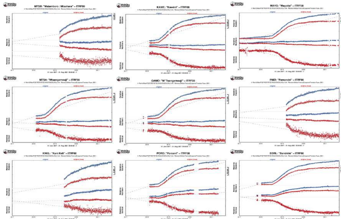
Figure 9 : Déplacements (en cm) enregistrés sur les 9 stations GPS localisées à Mayotte (MTSB, KAWI, MAYG, MTSA, GAMO, PMZI, KNKL, PORO, BDRL) entre le 1 er janvier 2017 et 31 août 2021 pour visualiser une longue série temporelle anté-crise. En bleu les données brutes, en rouge les données corrigées du mouvement de la plaque. Les stations sont présentées dans un ordre géographique ; du nord au sud (de haut en bas) et d'ouest en est (de gauche à droite). Post-traitement de ces données réalisé par l'IPGP (©OVPF-IPGP / REVOSIMA).
