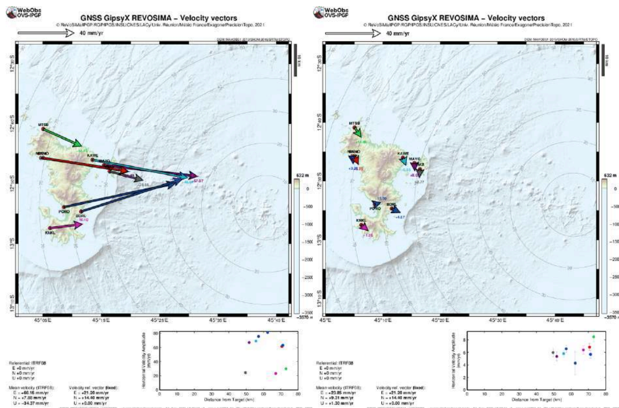
Figure 7 : Déplacements du sol enregistrés sur les stations GPS de Mayotte depuis le 1 er juillet 2018 (à gauche) et sur les derniers douze mois (à droite). Les déplacements horizontaux sont représentés sous forme vectorielle et les déplacements verticaux sont indiqués par les valeurs chiffrées en couleur. Post-traitement de ces données réalisé par l'IPGP (©OVPF-IPGP / REVOSIMA).
