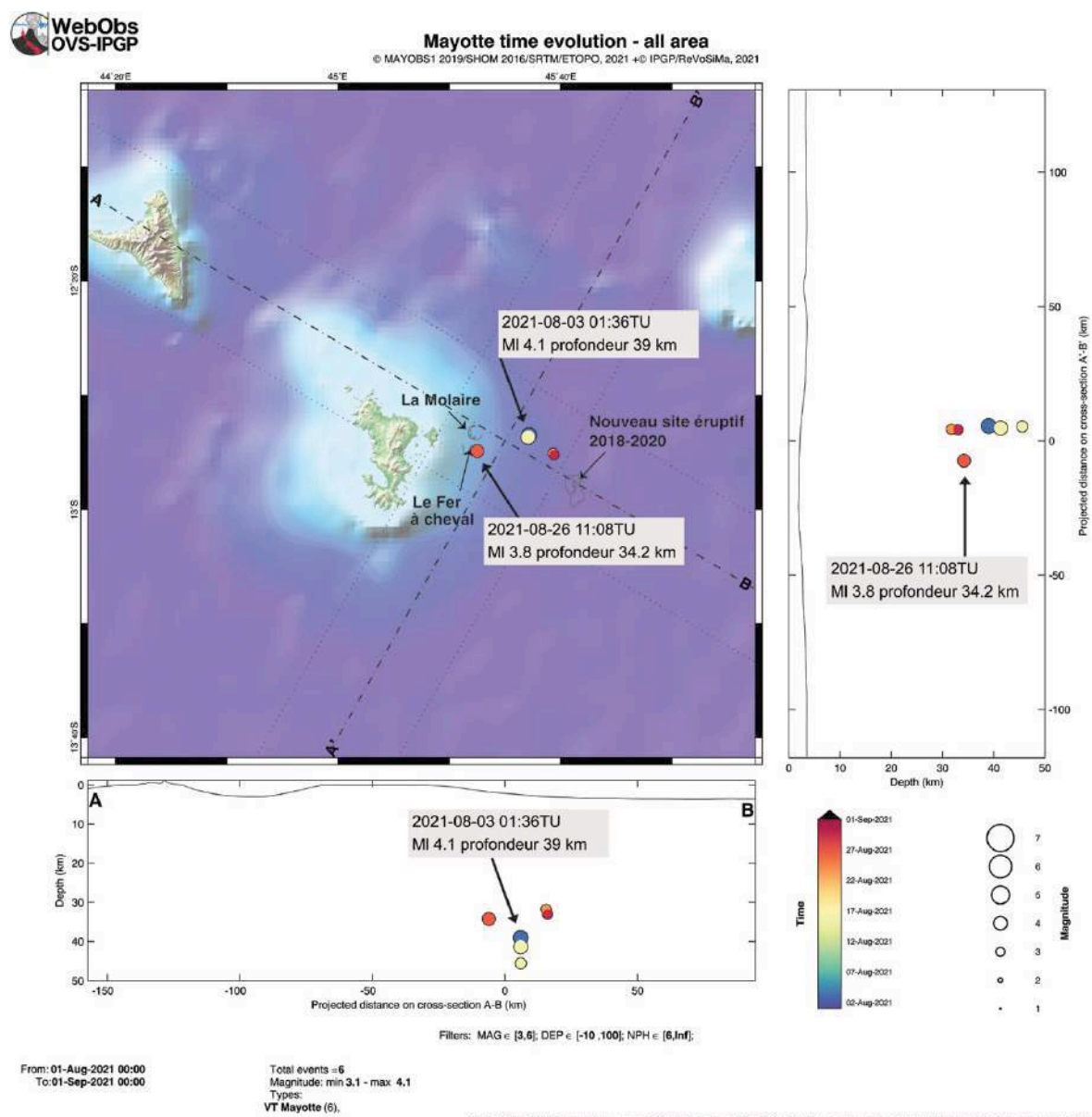
Figure 1c : Carte de localisation des épicentres ( \pm 5 km) des séismes volcano-tectoniques (VT) de magnitude M \geq 3 entre le 1 er et le 31 août 2021 enregistrés avec les réseaux sismiques de terre (IPGP-IFREMER-CNRS-BRGM-BCSF-RENASS, IPGS). Sont aussi représentées une projection des hypocentres des séismes le long de coupes transverses et axiales le long de la ride montrant la localisation estimée en profondeur (la précision varie entre \pm 5 km et \pm 15 km) des séismes en fonction de la magnitude (taille des symboles) et de la date (échelle temporelle de couleur). Les structures volcaniques de la zone dite de « La Molaire », du « Fer à cheval » sont indiquées en gris tout comme les coulées de lave du site éruptif. De nombreux points de sortie de panaches de fluides dans la colonne d'eau ont été identifiés dans la structure du Fer à Cheval avec une signature géochimique magmatique (voir section Géochimie des fluides). © OVPF-IPGP, BRGM, IFREMER, CNRS, BCSF-RENASS, IPGS / REVOSIMA).
