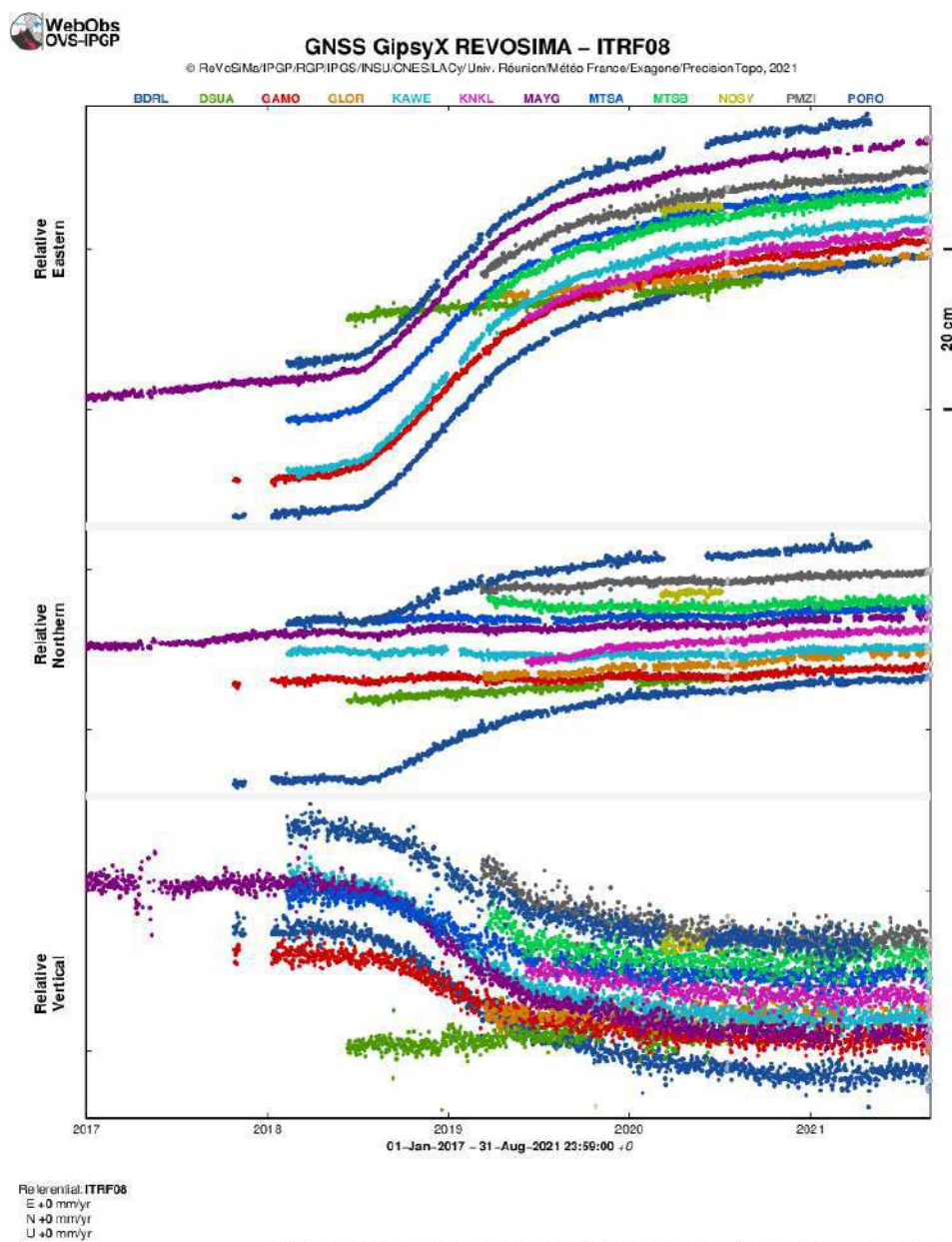
Figure 8 : Déplacements (en cm) enregistrés sur 9 stations GPS localisés à Mayotte (BDRL, GAMO, KAWE, KNKL, MAYG, MTSA, MTSB, PMZI, PORO), 1 station à Grande Glorieuse (GLOR) et 2 stations au nord de Madagascar à Diego Suarez (DSUA) et Nosy Be (NOSY) sur les composantes est (en haut), nord (au milieu) et vertical (en bas) entre le 1 er janvier 2017 et le 31 août 2021 pour visualiser une longue série temporelle anté-crise. Post-traitement de ces données réalisé par l'IPGP (©OVPF-IPGP / REVOSIMA).
