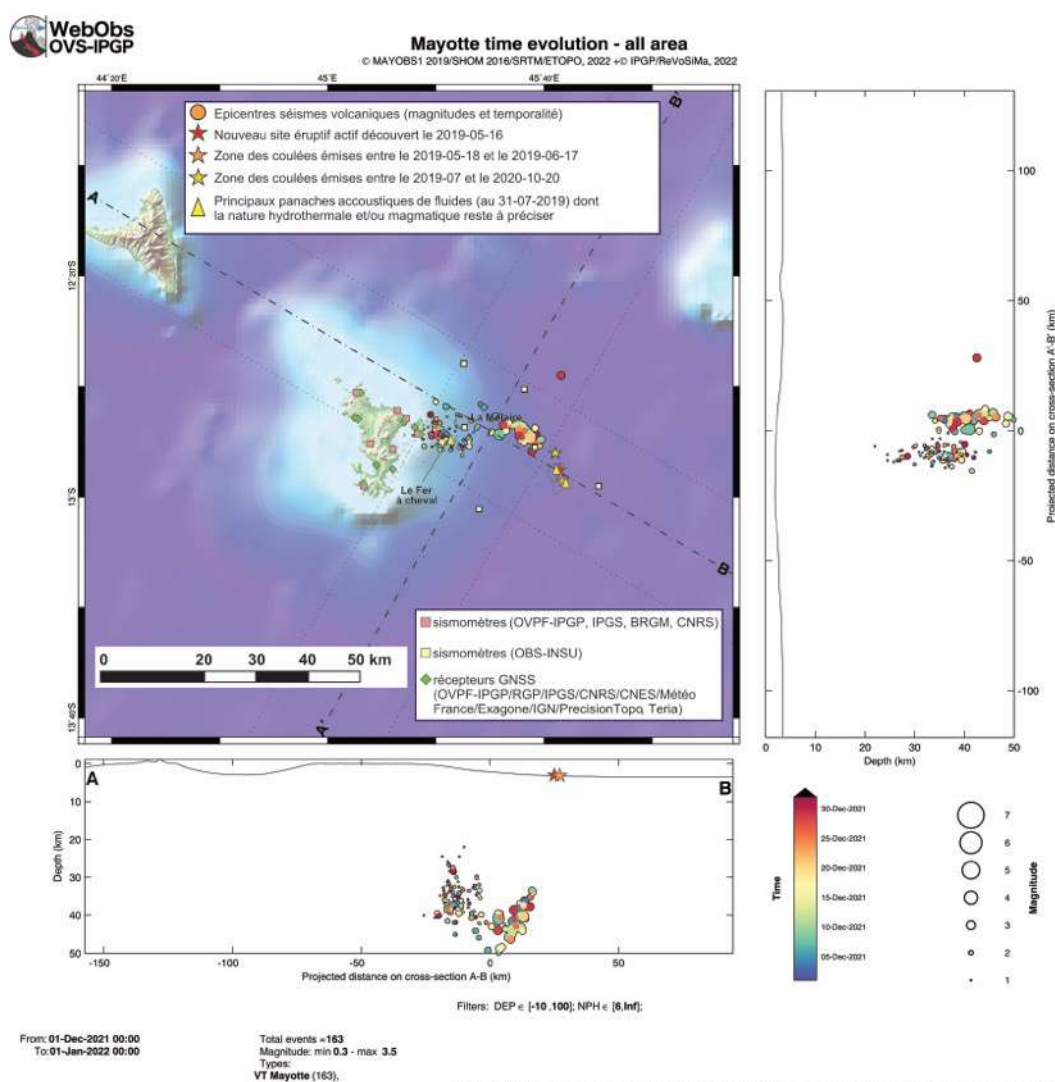
Figure 1a : Carte des épicentres ( \pm 5 km) des séismes volcano-tectoniques (VT) localisés avec les réseaux sismiques à terre (IPGP-IFREMER-CNRS-BRGM-BCSF-RENASS, IPGS) entre le 1 er et 31 décembre 2021 (échelle temporelle de couleur). Sont aussi représentées une projection des hypocentres des séismes le long de coupes transverses et axiales le long de la ride montrant la localisation estimée en profondeur (la précision varie entre \pm 5 km et \pm 15 km) des séismes en fonction de la magnitude (taille des symboles et de la date (échelle temporelle de couleur)). La localisation approximative des panaches acoustiques identifiés pendant les campagnes océanographiques (MD220-MAYOBS1, MD221-MAYOBS2, MD222-MAYOBS3, MD223-MAYOBS4, MAYOBS15, MAYOBS17) et dont la nature hydrothermale et/ou magmatique reste à préciser, est indiquée par des triangles jaunes, l'étoile rouge indique le site éruptif nouvellement identifié le 16 mai 2019, l'étoile orange la zone des coulées émises entre le 18/05/2019 et le 17/06/2019 et l'étoile jaune la zone des coulées émises entre juillet 2019 et le 18/01/2021. Les structures volcaniques de la zone dite de « La Couronne » sont indiquées en grisé tout comme les coulées de lave du site éruptif. Les stations sismiques du réseau terrestre, les sismomètres fond de mer (OBS) et les stations de positionnement par satellite GPS sont indiquées par des symboles (voir légende). (©OVPF-IPGP, BRGM, IFREMER, CNRS, BCSF-RENASS, IPGS / REVOSIMA).
