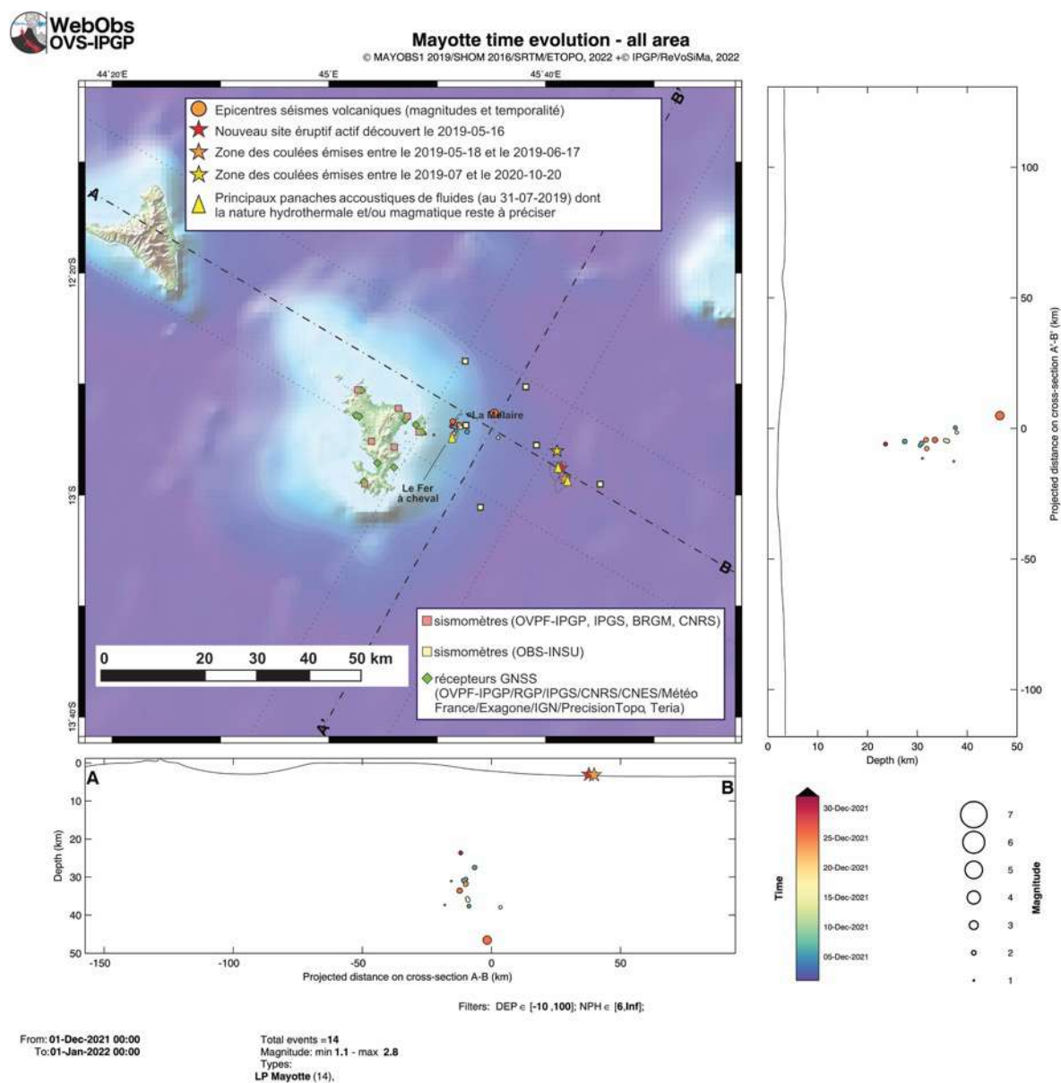
Figure 1b : Carte des épicentres ( \pm 5 km) des séismes longue période (LP) localisés avec les réseaux sismiques à terre (IPGP-IFREMER-CNRS-BRGM-BCSF-RENASS, IPGS) entre le 1 er et 31 décembre 2021 (échelle temporelle de couleur). Sont aussi représentées une projection des hypocentres des séismes le long de coupes transverses et axiales le long de la ride montrant la localisation estimée en profondeur (la précision varie entre \pm 5 km et \pm 15 km) des séismes en fonction de la magnitude (taille des symboles et de la date (échelle temporelle de couleur)). La localisation approximative des panaches acoustiques identifiés pendant les campagnes océanographiques (MD220-MAYOBS1, MD221-MAYOBS2, MD222-MAYOBS3, MD223-MAYOBS4, MAYOBS15, MAYOBS17) et dont la nature hydrothermale et/ou magmatique reste à préciser, est indiquée par des triangles jaunes, l'étoile rouge indique le site éruptif nouvellement identifié le 16 mai 2019, l'étoile orange la zone des coulées émises entre le 18/05/2019 et le 17/06/2019 et l'étoile jaune la zone des coulées émises entre juillet 2019 et le 18/01/2021. Les structures volcaniques de la zone dite de « La Molaire » sont indiquées en grisé tout comme les coulées de lave du site éruptif. Les stations sismiques du réseau terrestre, les sismomètres fond de mer (OBS) et les stations de positionnement par satellite GPS sont indiquées par des symboles (voir légende). (©OVPF-IPGP, BRGM, IFREMER, CNRS, BCSF-RENASS, IPGS / REVOSIMA).
