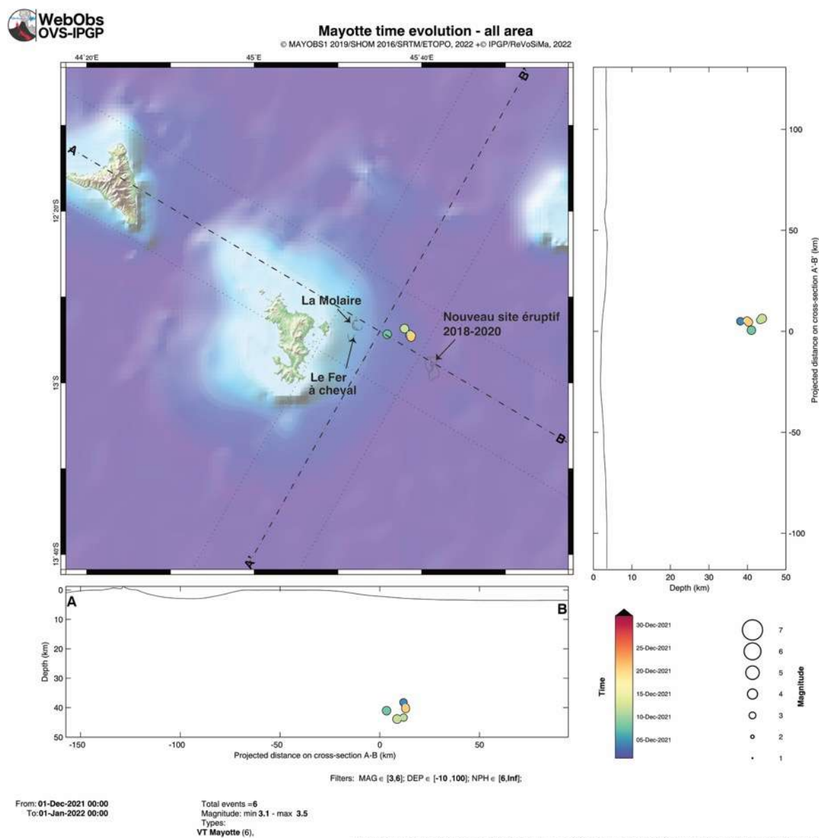
Figure 1c : Carte de localisation des épicentres ( \pm 5 km) des séismes volcano-tectoniques (VT) de magnitude M \geq 3 entre le 1 er et le 31 décembre 2021 enregistrés avec les réseaux sismiques à terre (IPGP-IFREMER-CNRS-BRGM-BCSF-RENASS, IPGS). Sont aussi représentées une projection des hypocentres des séismes le long de coupes transverses et axiales le long de la ride montrant la localisation estimée en profondeur (la précision varie entre \pm 5 km et \pm 15 km) des séismes en fonction de la magnitude (taille des symboles) et de la date (échelle temporelle de couleur). Les structures volcaniques de la zone dite de « La Molaire », du « Fer à cheval » sont indiquées en grisé tout comme les coulées de lave du site éruptif. De nombreux points de sortie de panaches de fluides dans la colonne d'eau ont été identifiés dans la structure du Fer à Cheval avec une signature géochimique magmatique (voir section Géochimie des fluides). © OVPF-IPGP, BRGM, IFREMER, CNRS, BCSF-RENASS, IPGS / REVOSIMA).
